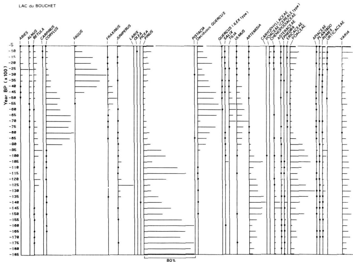
Résumé du diagramme pollinique du Lac du Bouchet (DE BEAULIEU et al. , 1984).
