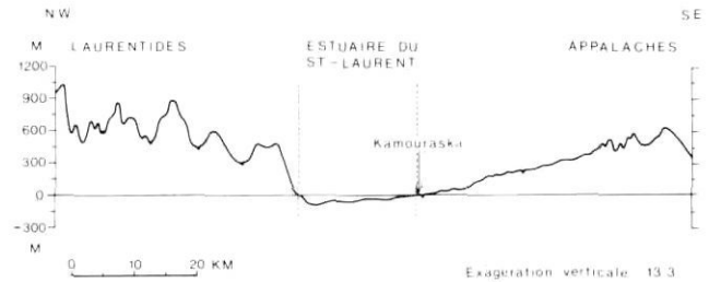
FIGURE 4. Profil topographique et bathymétrique transversal du moyen estuaire du Saint-Laurent, à Kamouraska.
