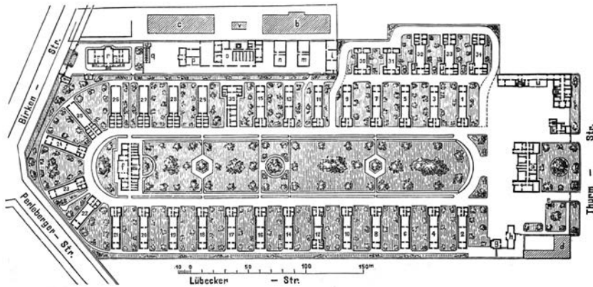
1. – 34. Baracken. 35. Isolirbaracke. a. Künftiges Verwaltungsgebäude. b. Künftige Kochküche. c. Künftige Waschküche. d. Feuerwehrestelle. e. Abort. f. Operationshaus. g. Kleiderschuppen. h. Schuppen. k. Pförtner. l. Werkstatt. m. n. Schuppen. o. Kesselhaus. p. Desinfectionshaus. q. Stall für Versuchsthiere. r. Leichenhalle. s. Abort. t. Wage. v. Künftiger Wagenschuppen. w. Pförtner an der Birkenstraße.
