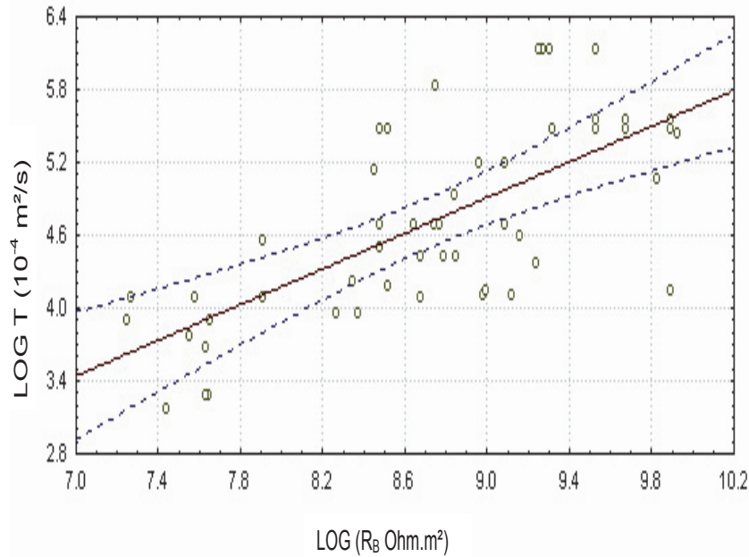
Figure 7 Diagramme de régression Log-Log entre les transmissivités ( T_{mes} ) et les résistances transversales des lentilles perméables saturées ( R_p ). Log-Log regression diagram between measured transmissivities ( T_{mes} ) and transverse resistances of the pervious layers ( R_p ).
