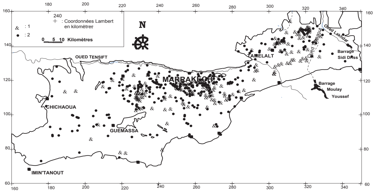
Figure 2 Localisation des ouvrages testés par pompages d'essai. 1 : Forage; 2 : Puits à grand diamètre. Location of the tested wells using pumping tests. 1: Borehole; 2: Large diameter well.
