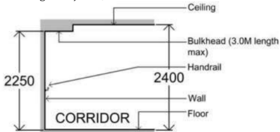
Gambar 3.3 : Bagian Koridor yang menunjukkan ketinggian langit-langit minimum
