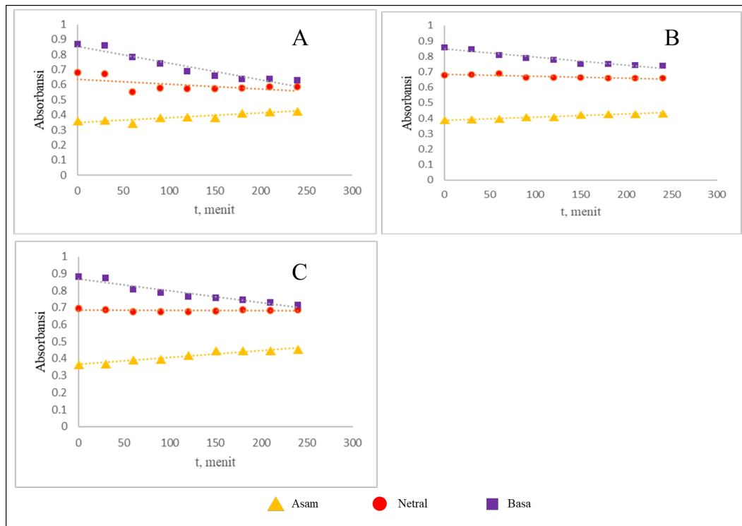
GAMBAR 5. Absorbansi produk hasil metilasi brazilein pada suhu a) 50 °C, b) 60 °C, dan c) 70 °C
