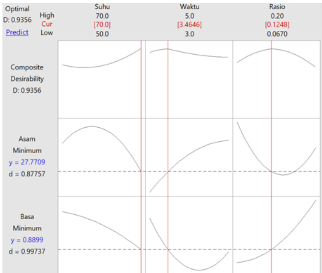
GAMBAR 9. Kondisi optimum reaksi metilasi brazilein
