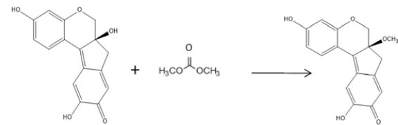
GAMBAR 2. Mekanisme reaksi antara brazilein dengan dimetil karbonat (Ulma dkk. 2018).
