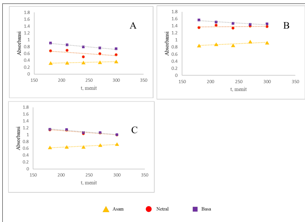
GAMBAR 6. Absorbansi produk hasil metilasi brazilein pada rasio pereaksi a) 0,2 b) 0,1 dan c) 0,067
