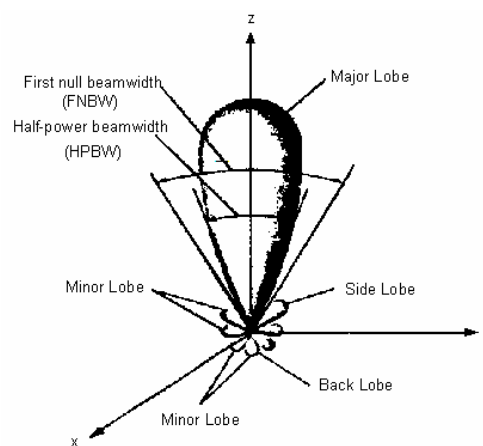
Gambar 1 Pola Radiasi (Sumber: [1] : 31)
