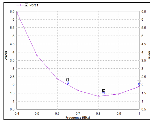
Gambar 7. Grafik VSWR
