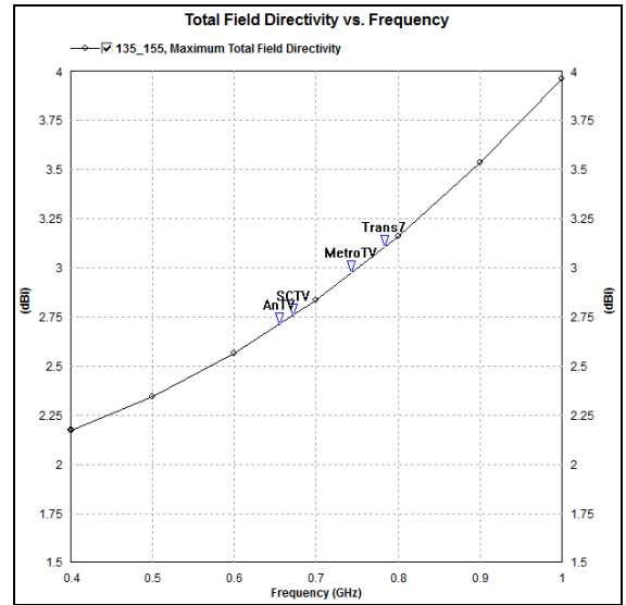
Gambar 11. Grafik Directivity
