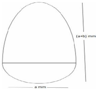
Gambar 4 Dimensi Antena Egg
