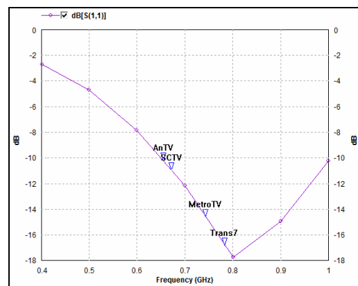
Gambar 8. Grafik Return Loss
