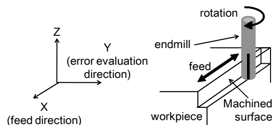
Fig. 1 Side-milling
