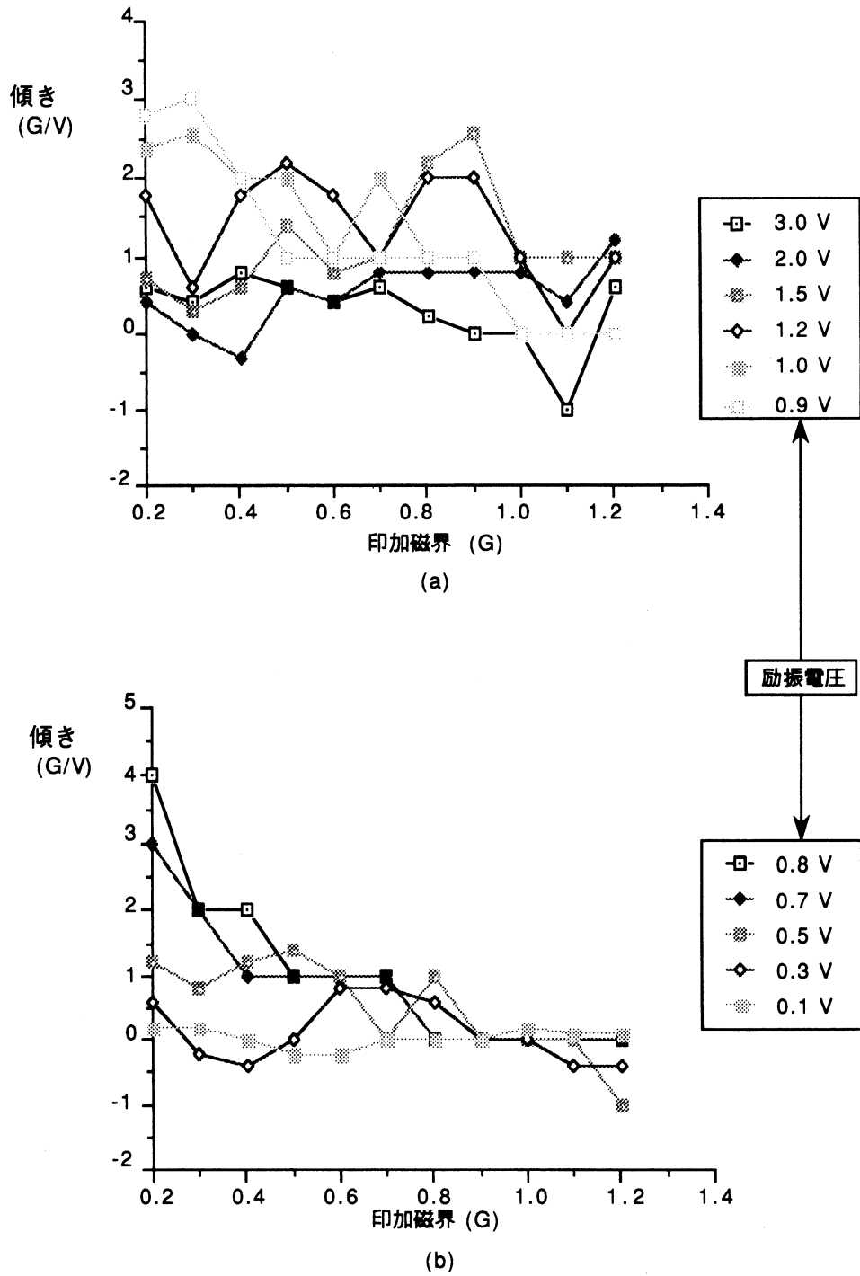
Fig. 4-2-2 出力電圧の変化 (傾き)
