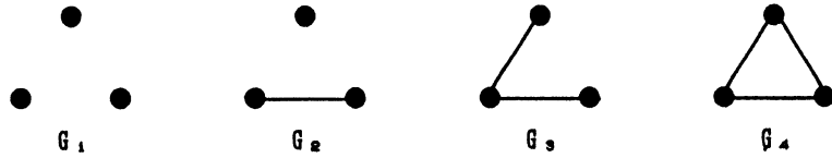
図4 G(3)のグラフ
