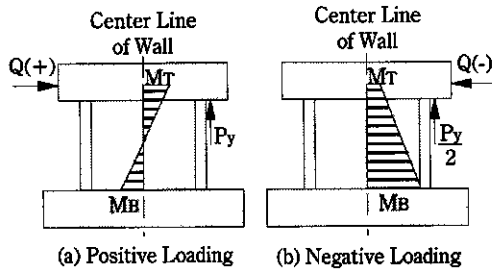
Fig. 4 Moment Distributions
