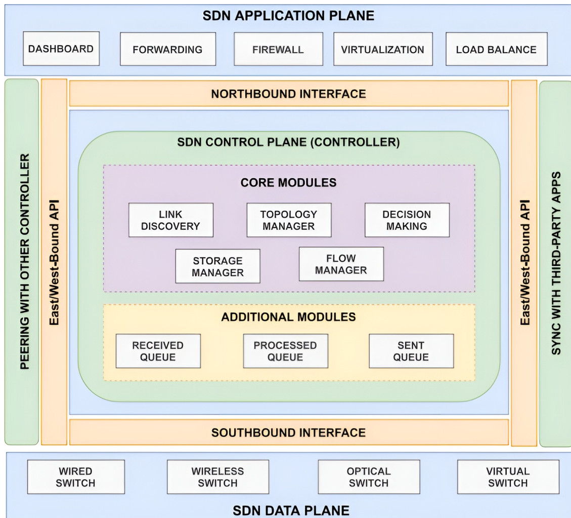
Figura 2.7: Arquitectura genérica de controlador SDN [44]
