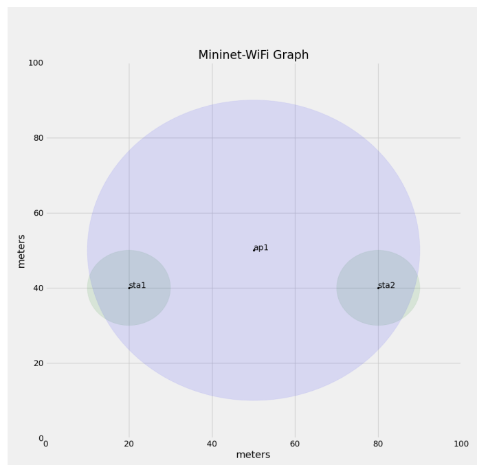
Figura 3.7: Topología básica haciendo uso del UserAP (BOFUSS)
