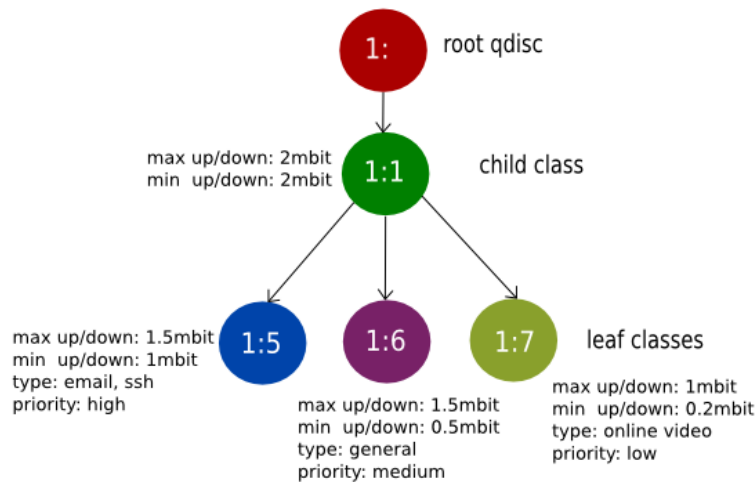
Figura 2.20: Mecanismo de calidad de servicio implementado con clases y sub-clases [60]
