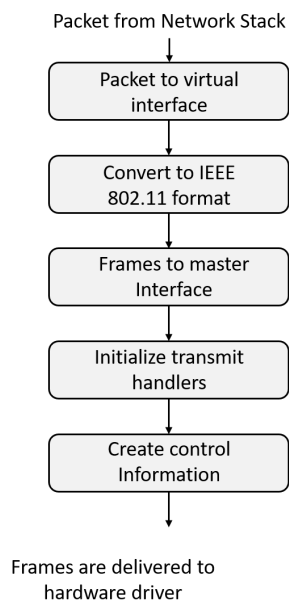
Figura 2.22: Pipeline de transmisión del módulo mac80211_hwsim [64]
