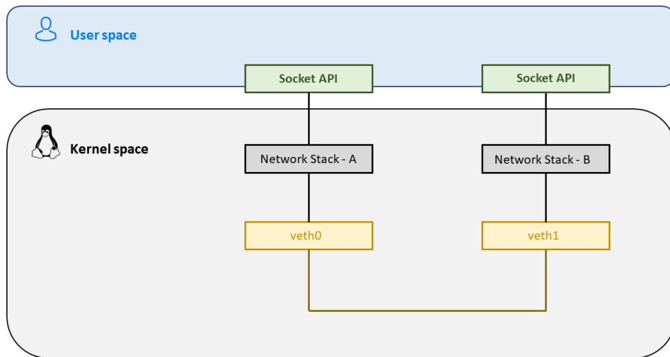
Figura 2.21: Enlace entre interfaces Veth separadas en dos Network Namespaces [18]
