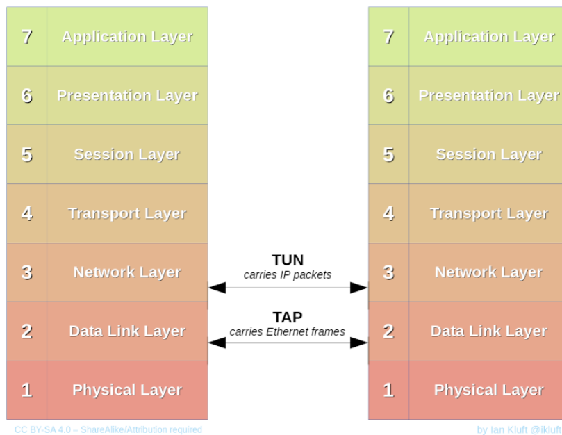
Figura 2.18: Diagrama de funcionamiento de las interfaces virtuales TUN/TAP [56]
