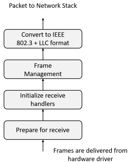
Figura 2.23: Pipeline de recepción del módulo mac80211_hwsim [64]
