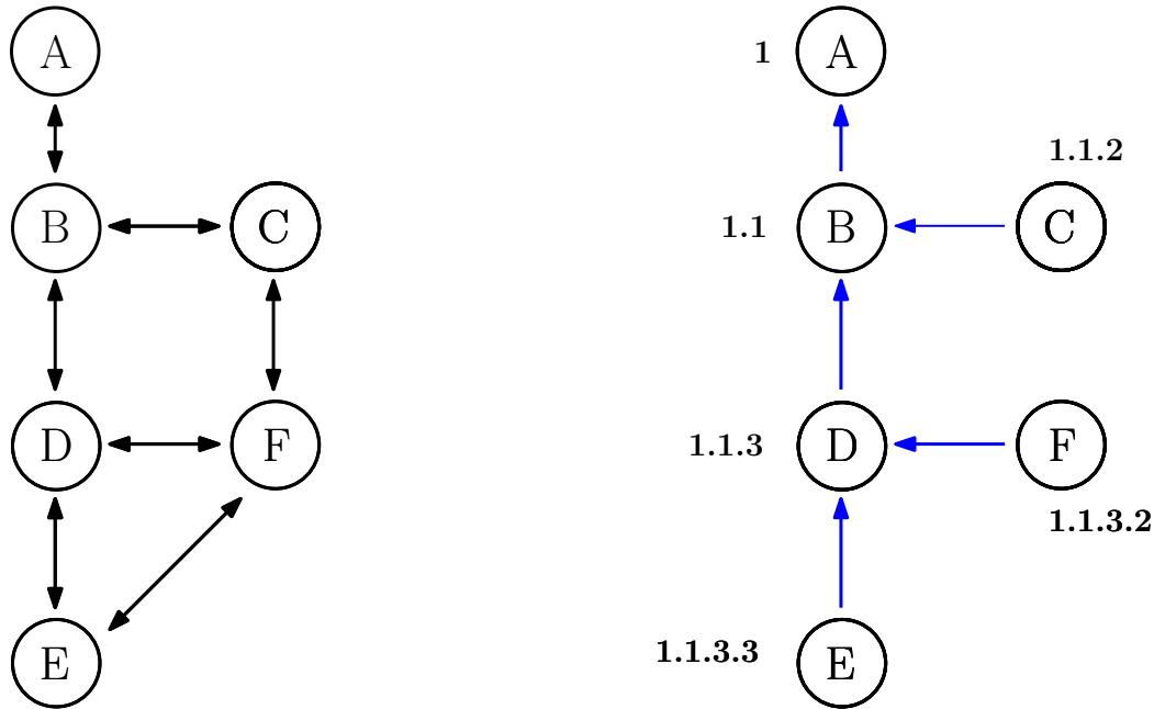
Figura 4.22: Establecimiento de la topología lógica
