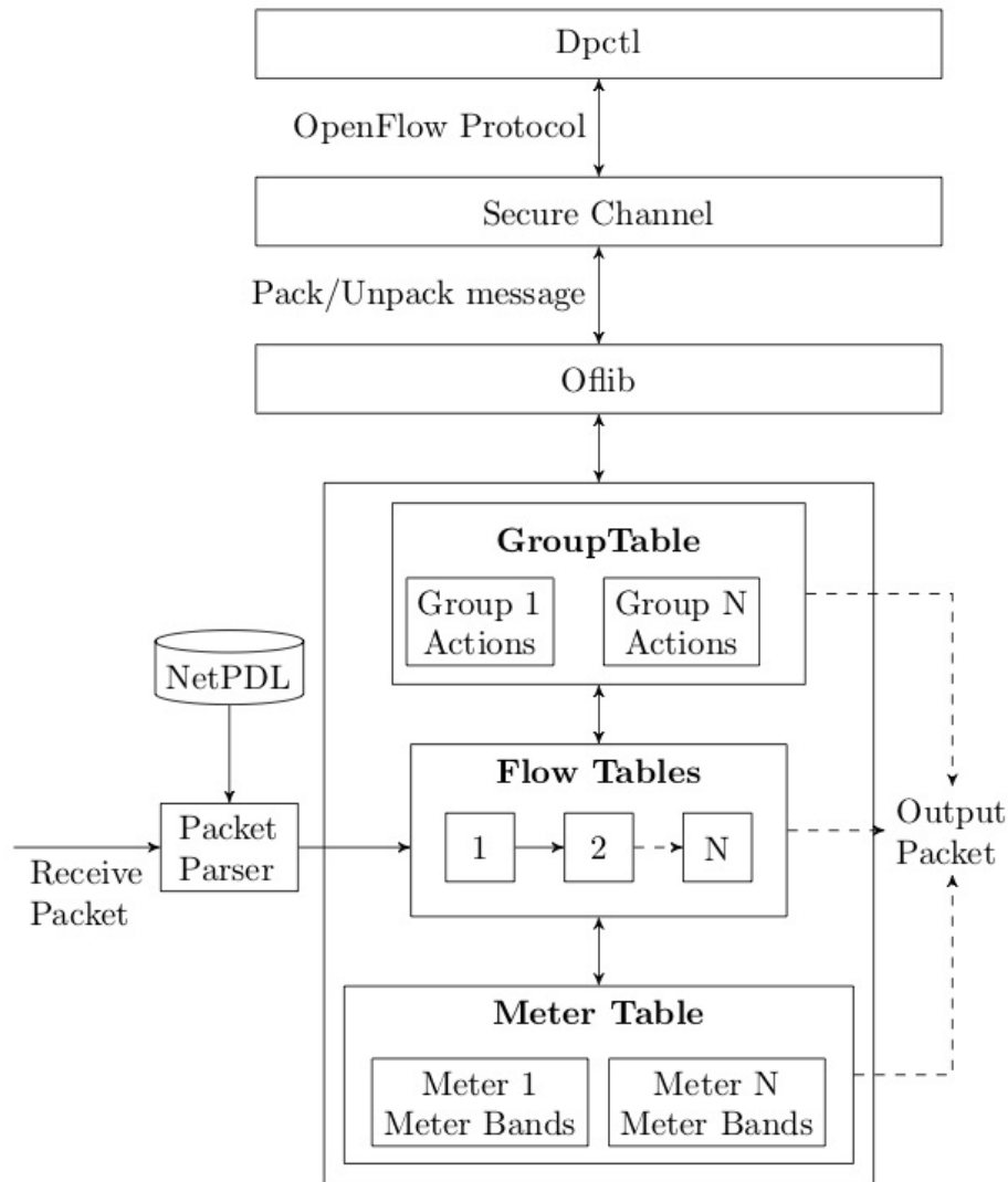
Figura 2.13: Arquitectura del BOFUSS [43]
