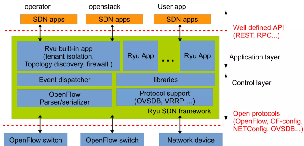
Figura 2.8: Arquitectura del controlador SDN RYU [47]
