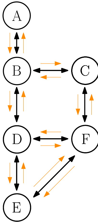
Figura 4.12: Intercambio de mensajes de tipo Hello en la topología básica
