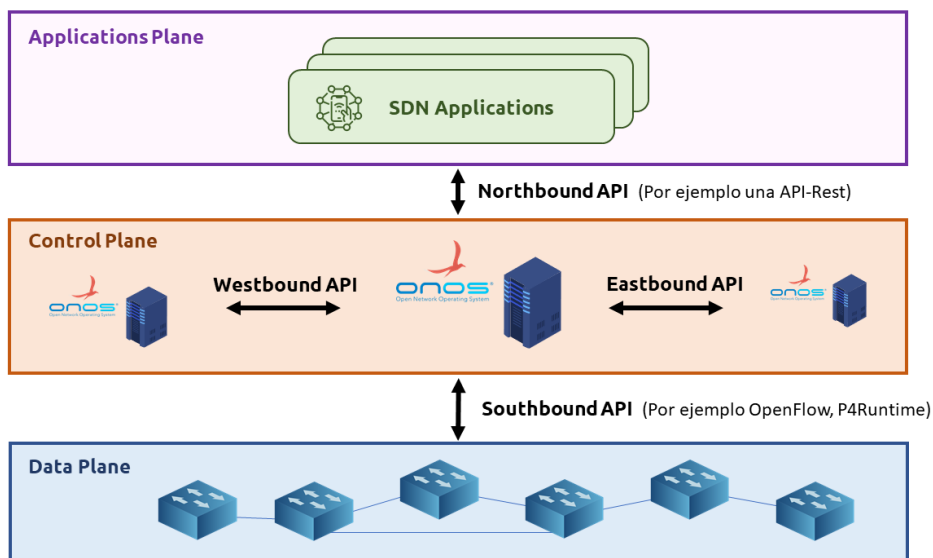
Figura 2.5: Arquitectura típica SDN [18]
