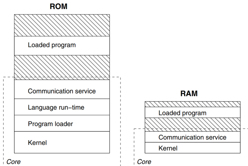
Figura 2.33: Gestión de la memoria en un sistema con Contiki OS [68]
