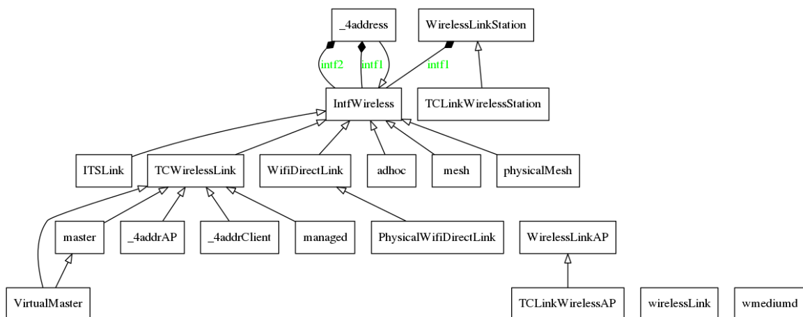
Figura 2.32: UML de clases de tipo Interfaz.
