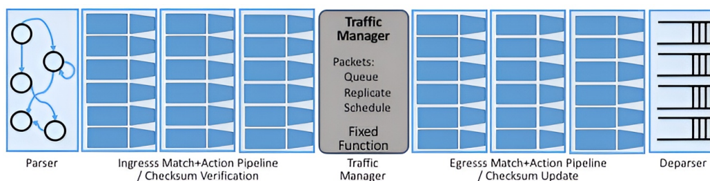
Figura 2.10: Arquitectura genérica de un softswitch SDN [51]
