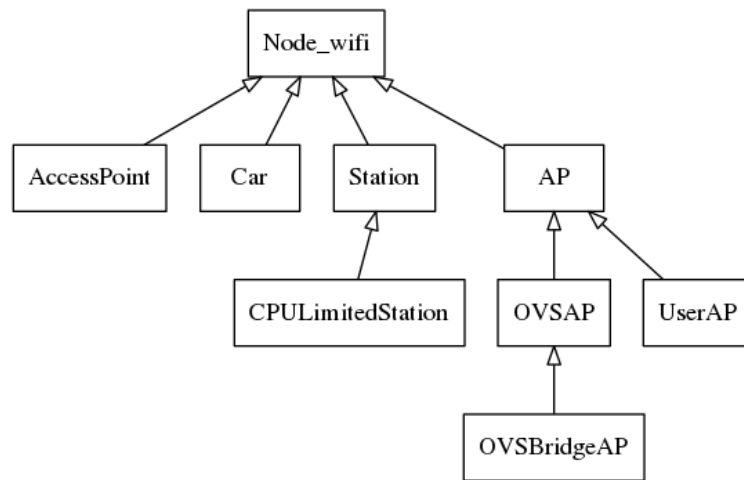
Figura 2.31: UML de clases de tipo Nodo.
