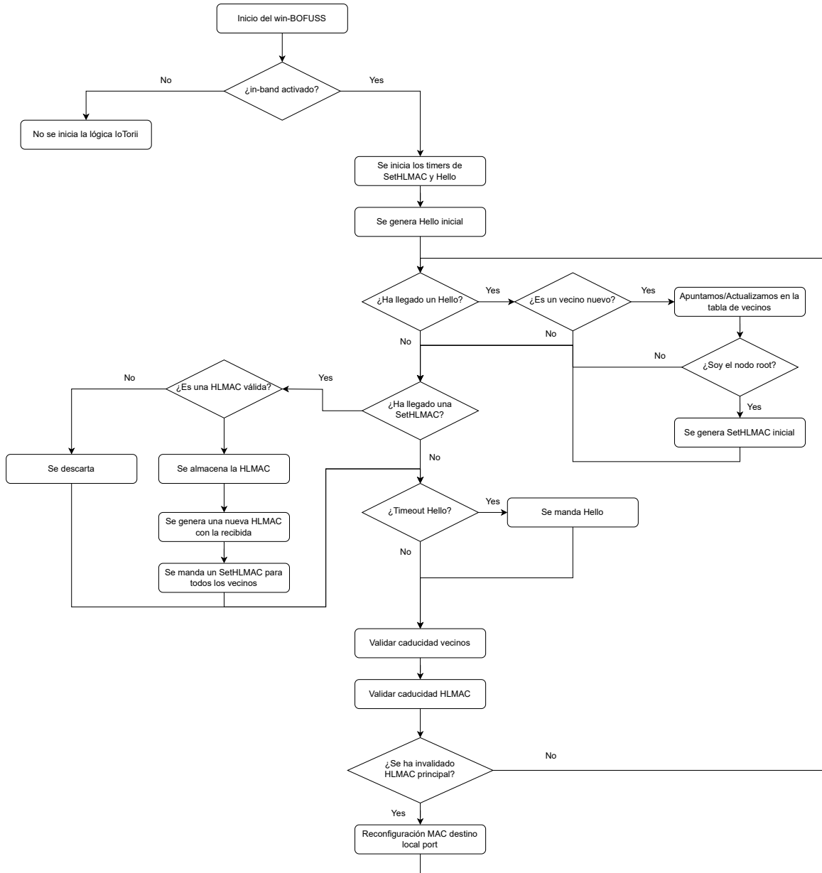
Figura 4.8: Diagrama de flujo de la operativa del protocolo IoTarii en el software switch BOFUSS
