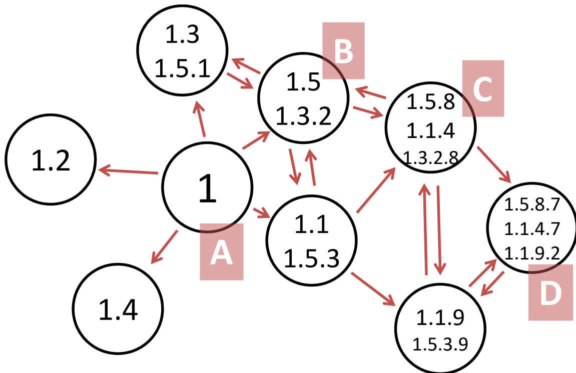
Figura 3.1: Operativa del protocolo de IoTarii [71]
