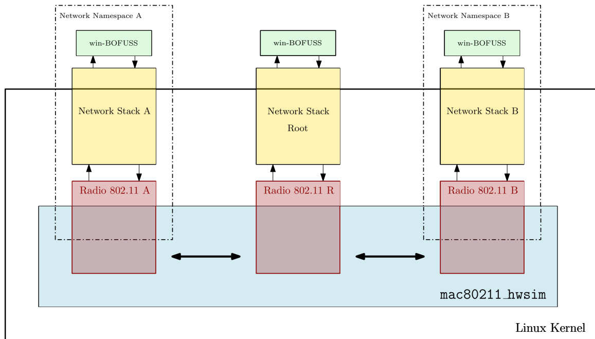
Figura 4.9: Entorno de validación haciendo uso del módulo del kernel mac80211_hwsim
