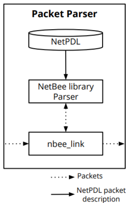
Figura 2.14: Parseador de paquetes del BOFUSS [43]
