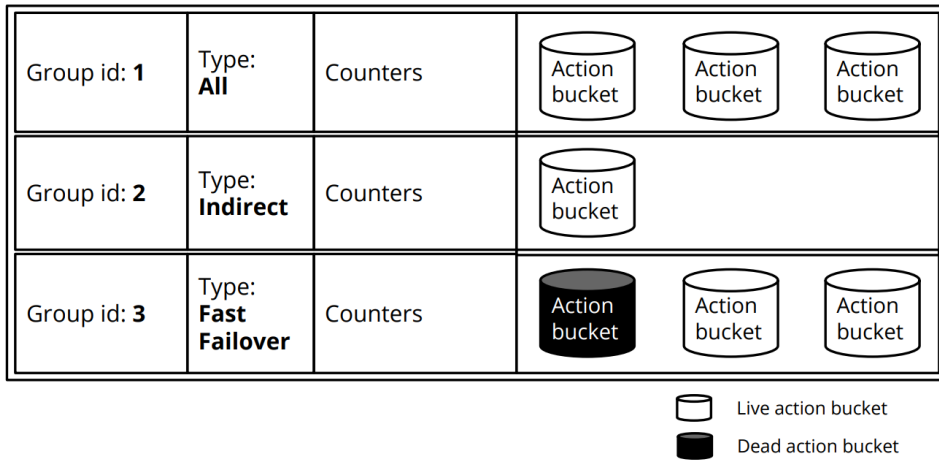
Figura 2.15: Estructura de las Group tables del BOFUSS [43]
