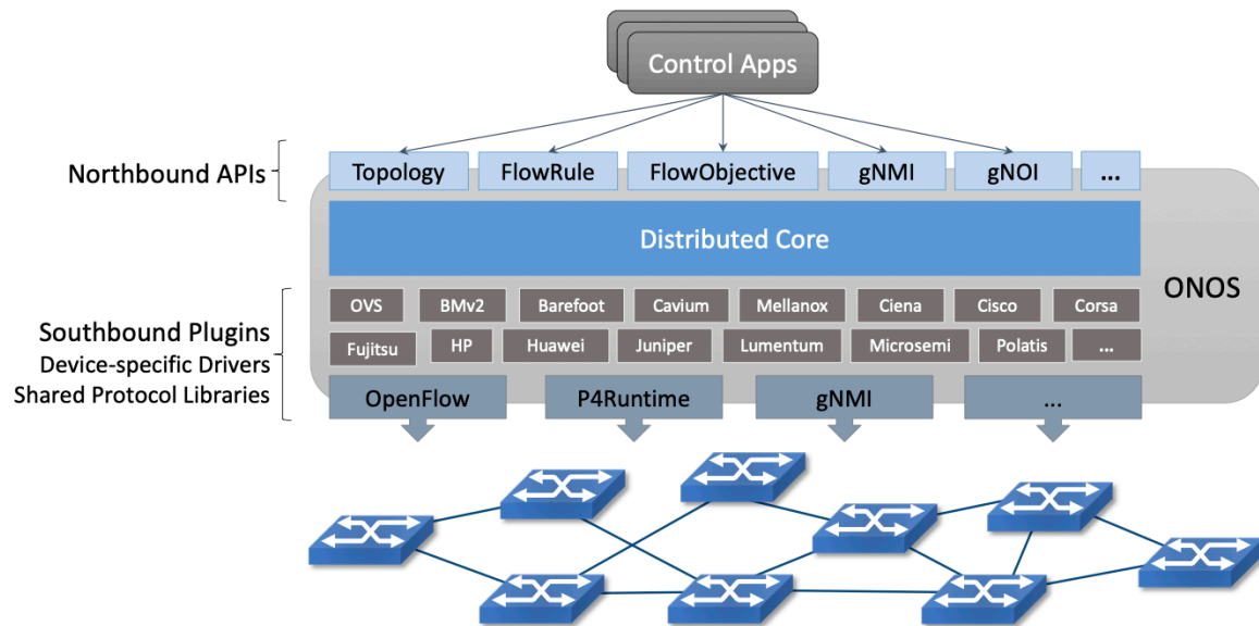
Figura 2.9: Arquitectura del controlador SDN onos [50]
