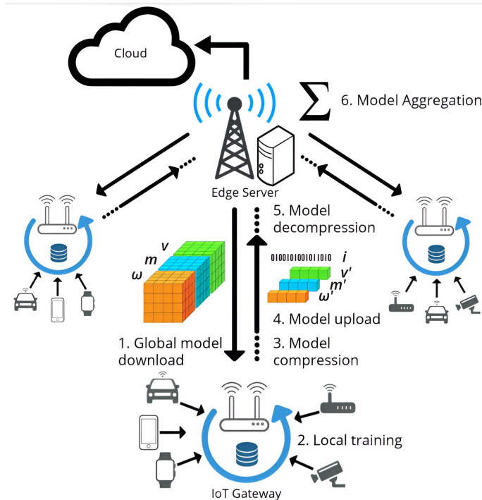
Figura 2.2: Esquema genérico de un sistema FL [33]
