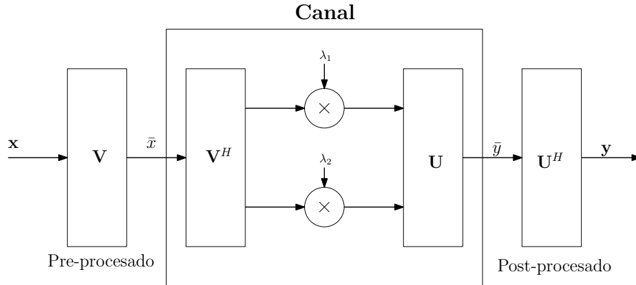
Figura 2.1: Descomposición genérica de un canal MIMO en subcanales paralelos
