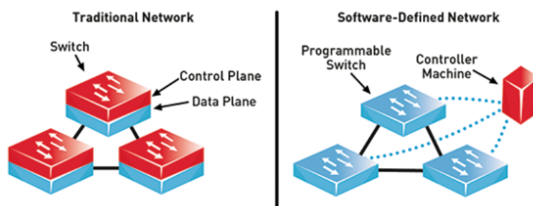
Figura 1.3: Paradigma en las redes SDN [18]
