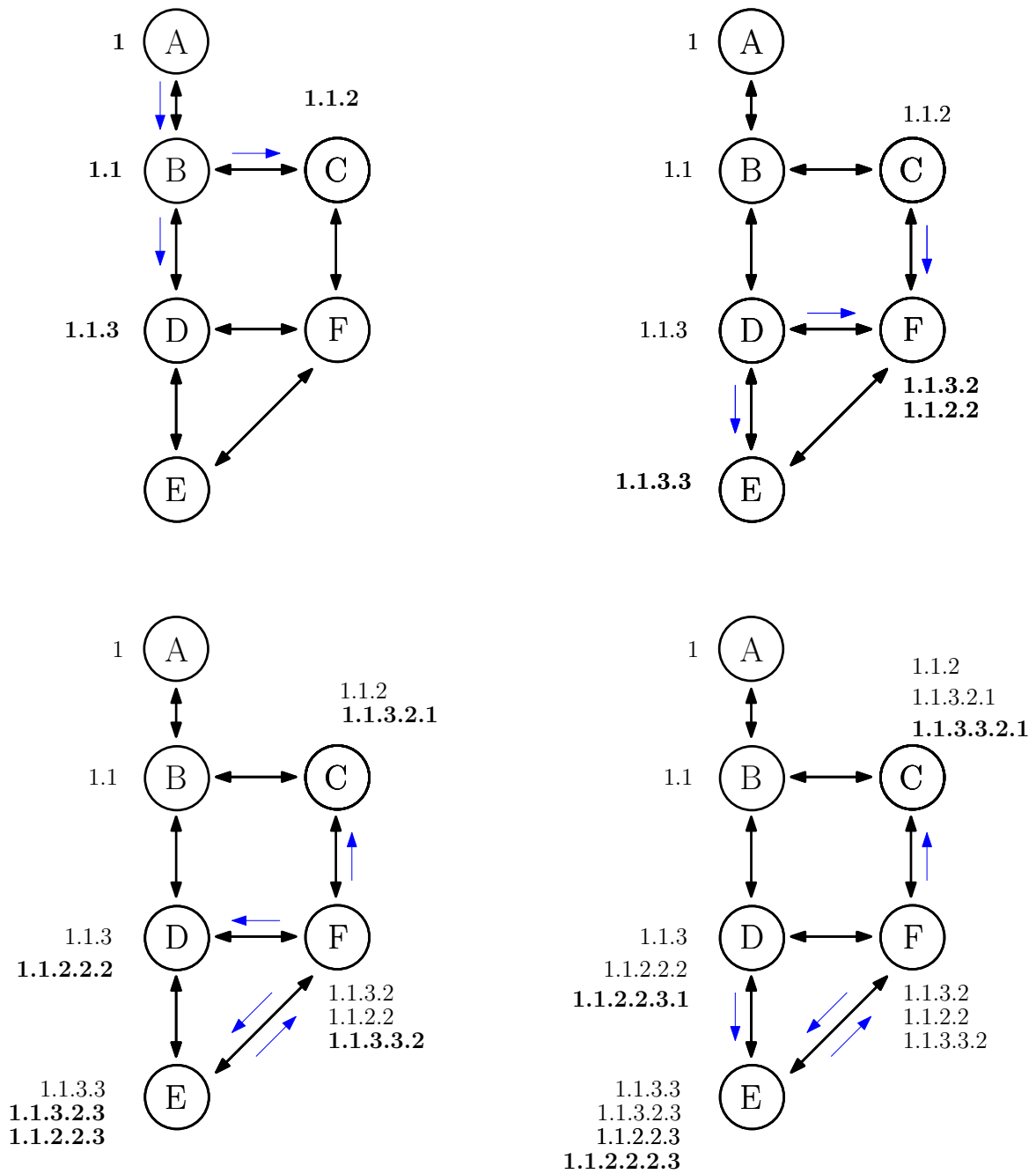
Figura 4.20: Proceso de difusión de mensajes de tipo SetHLMAC en la topología básica
