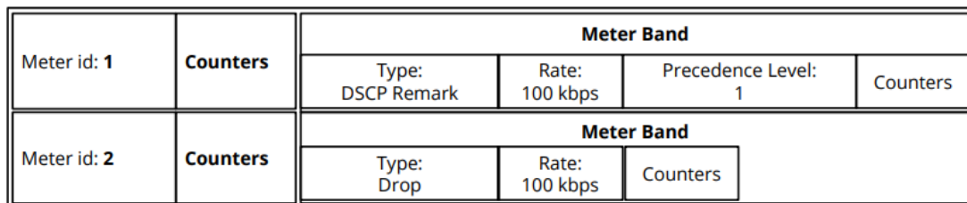
Figura 2.16: Estructura de las Meter tables del BOFUSS [43]
