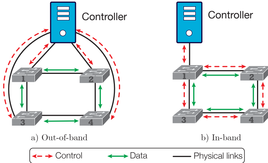
Figura 1.4: Paradigma control en las redes SDN [19]
