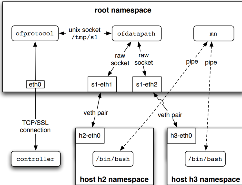
Figura 2.24: Arquitectura de Mininet [66]
