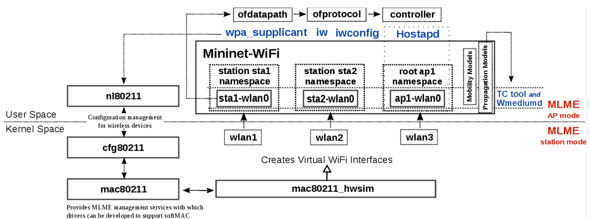
Figura 2.30: Arquitectura básica de Mininet-WiFi [67]
