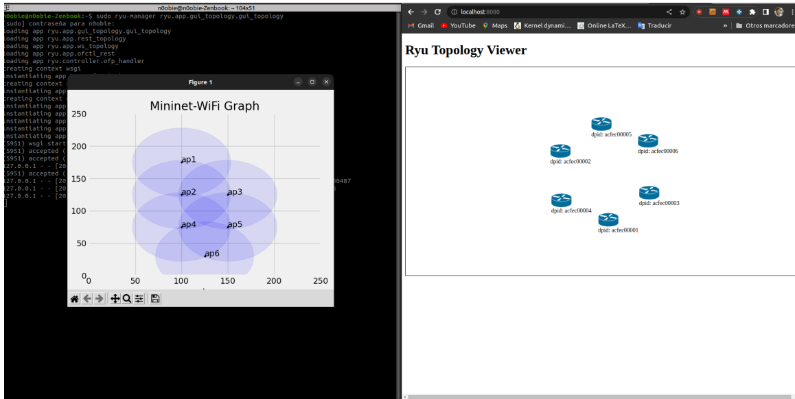
Figura 4.25: Descubrimiento topológico llevado a cabo por Ryu
