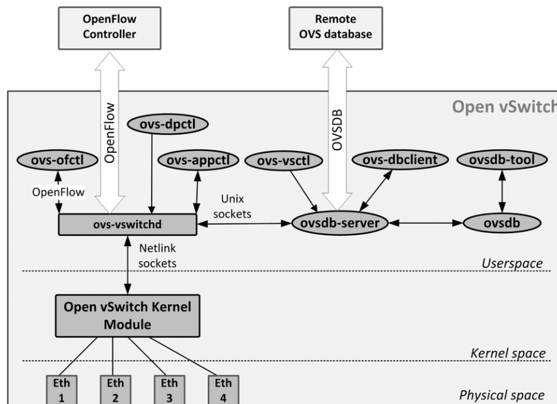
Figura 2.11: Arquitectura del OvS [53]
