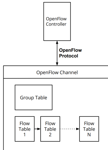
Figura 2.6: Arquitectura básica de agente OpenFlow [43]
