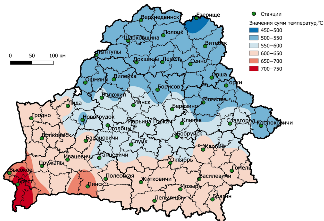
Рис. 1. Распределение сумм температур (°С) осеннего периода на территории Беларуси за 2000–2020 гг.
