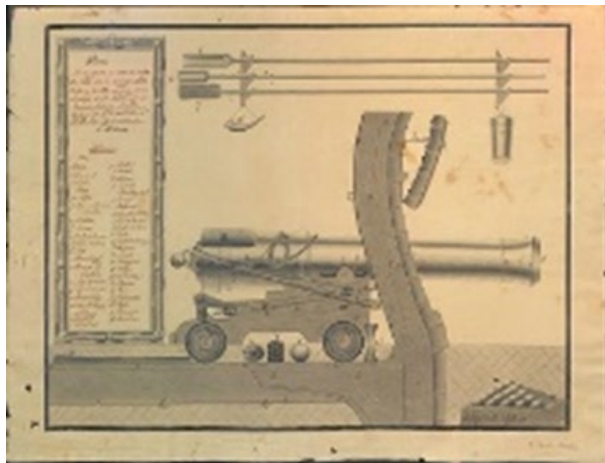
Ilustración 20 Dibujo de piezas de artillería realizadas por el alumno Francisco Galves González en 1853 Fuente: AHUS Caja 6
