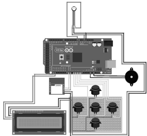
Gambar 7. Rangkaian sistem pengaturan Deteksi Target Heart rate (THR) pada Cardio Exercise Berbasis Metode Karvonen
