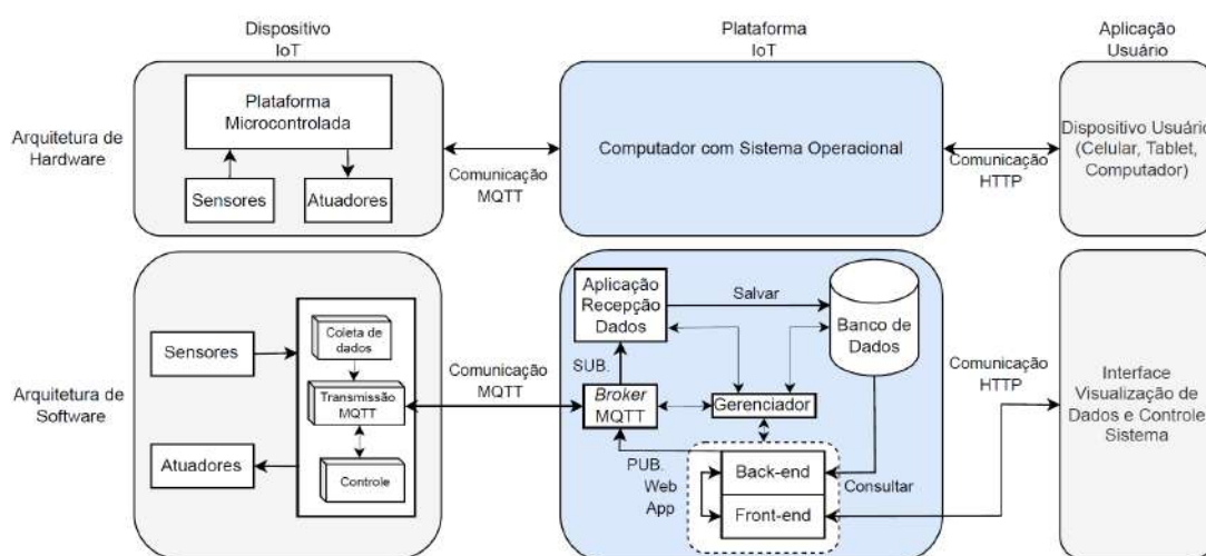
Figura 1: Arquitetura de Hardware e Software da Plataforma IoT
