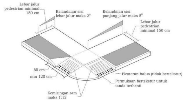
2.4 Gambar dimensi jangkauan
