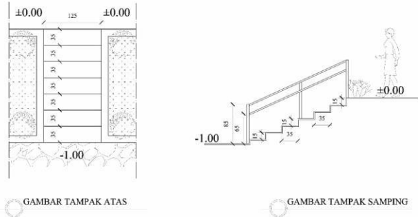
Gambar 4.8. Rekomendasi Dimensi
