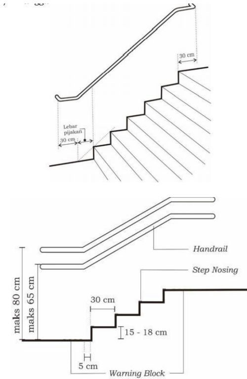
2.7. Gambar Tangga
