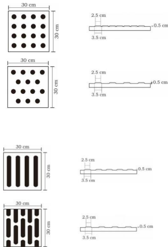
2.5. Pola Jalur pemandu
