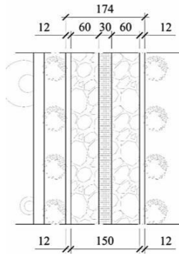
4.2. Dimensi jalan
