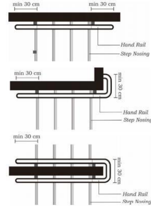
2.8. Gambar ukuran anak tangga
