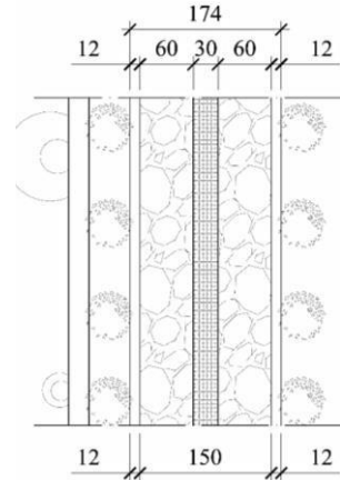
4.3. Gambar Dimensi Jalan
