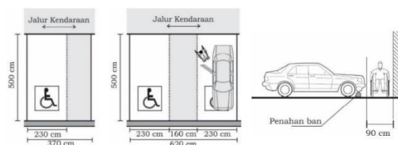
2.11. Gambar dimensi jalur difabel
