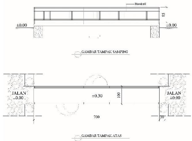
4.11. Gambar Layout Jembatan type B
