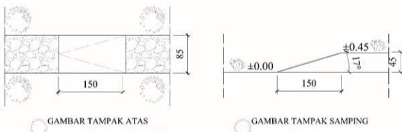
4.6. Gambar Layout
