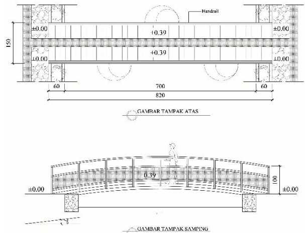
4.12. Gambar Rekomendasi Jembatan
