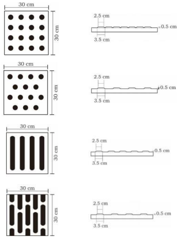
Gambar 4.4. Gambar Pola Jalur pemandu
