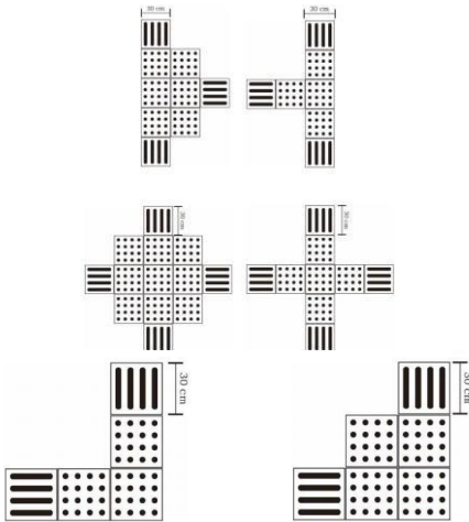
2.5. Gambar pola ubin pada jalur pedestrian
