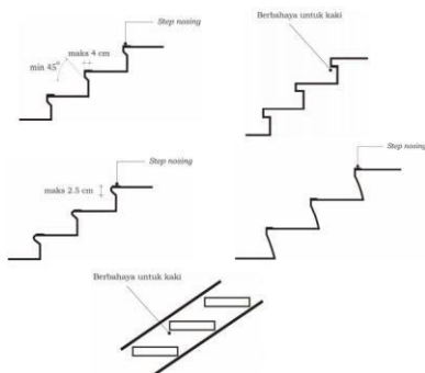
2.7. Gambar Tangga
