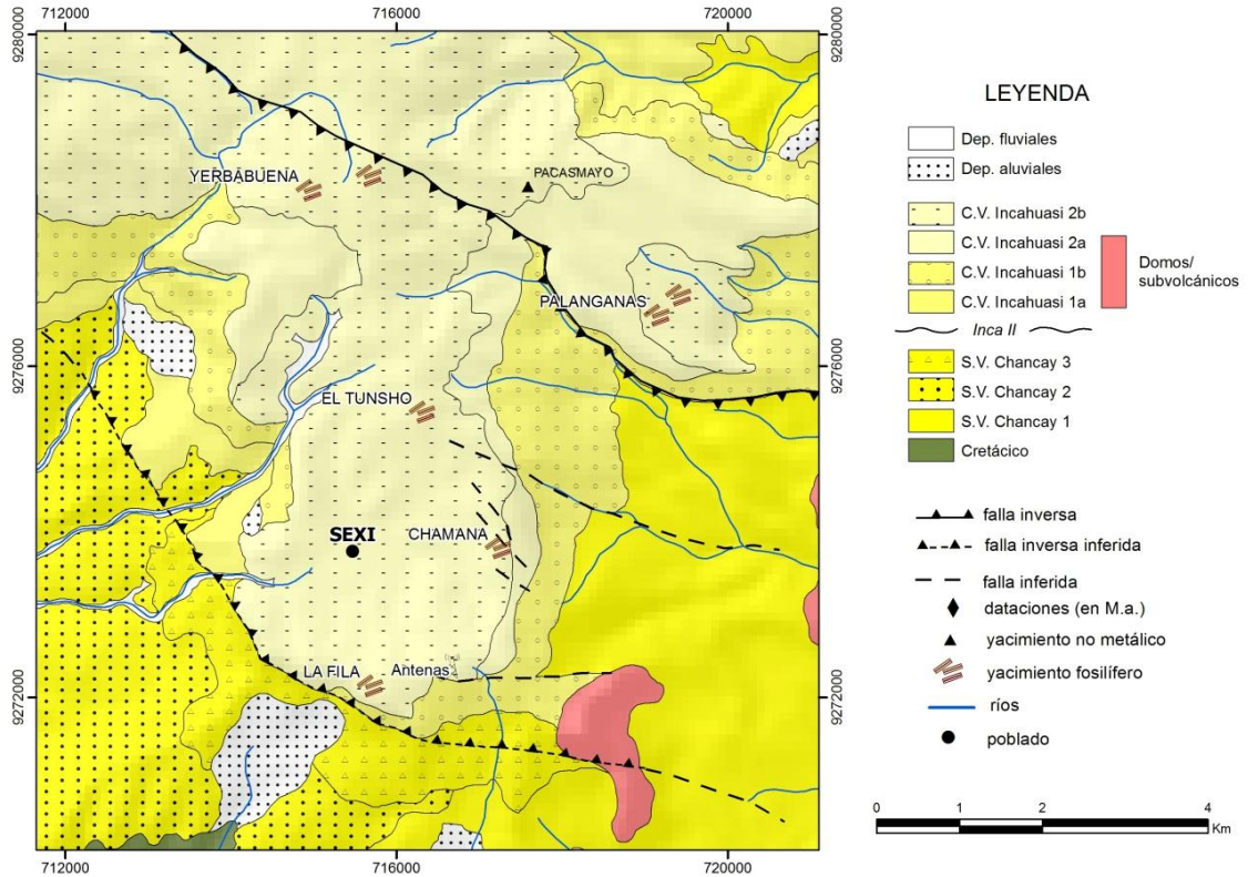
Figura 3.- Mapa geológico local del área de estudio
