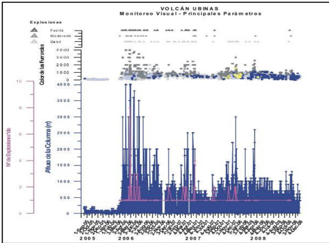
Figura 9. Altura y coloración de la pluma volcánica, así como número de explosiones, correspondientes a los años 2005, 2006, 2007 y 2008.
