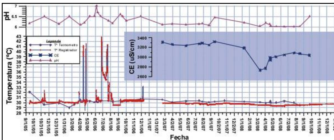
Figura 6. Parámetros fisicoquímicos registrados en la fuente UBT entre los años 2005 y 2008.
