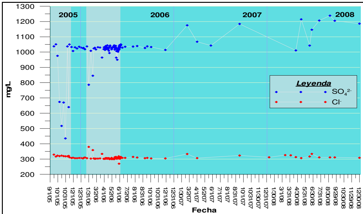
Figura 7. Gráfica de las concentraciones de aniones mayoritarios en la fuente UBT.
