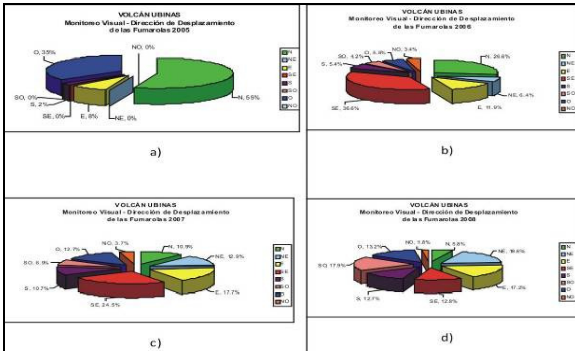
Figura 10. Porcentaje de desplazamiento de la pluma volcánica, entre los años 2005 y 2008.
