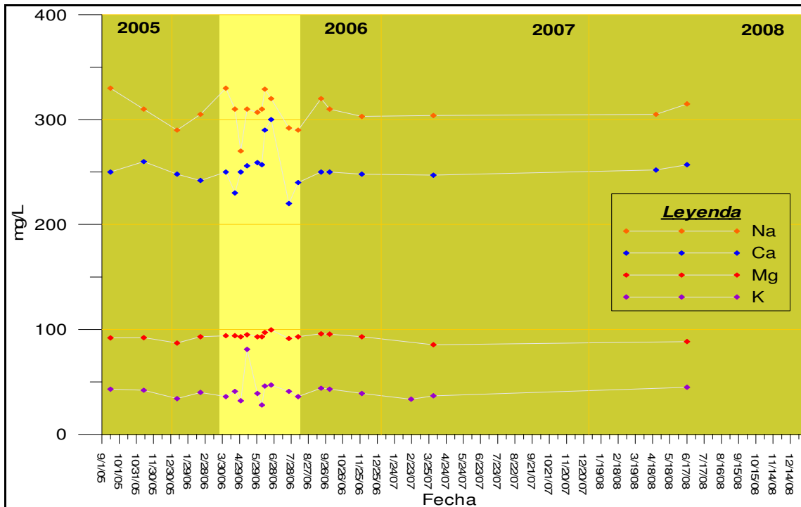
Figura 8. Gráfica de las concentraciones de cationes mayoritarios en la fuente UBT, años 2005 a 2008.
