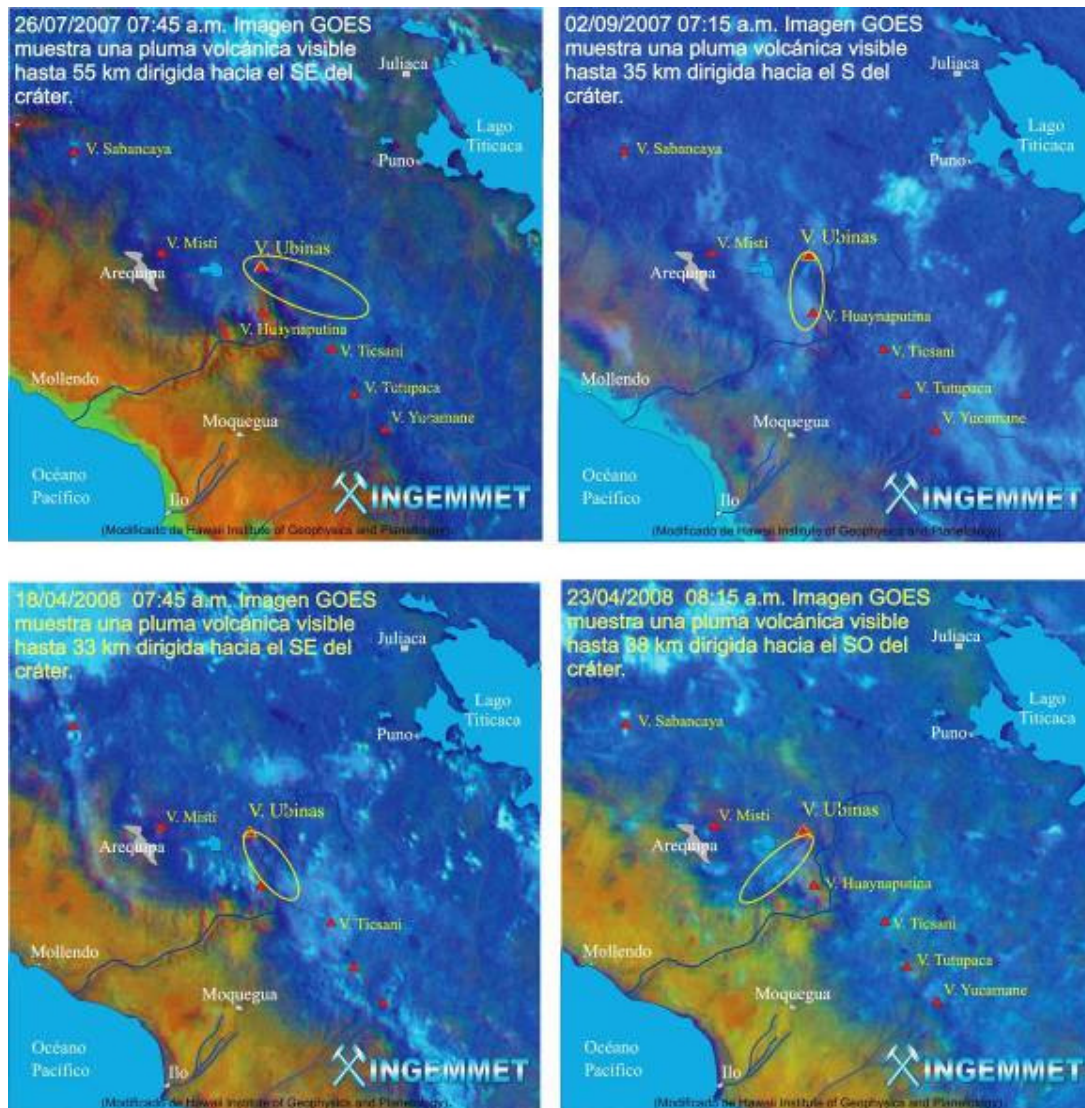
Figura 15. Imágenes de satélite GOES que muestran la dispersión de cenizas luego de las explosiones registradas los días 26 de julio y 2 de setiembre del 2007, así como los días 18 y 23 de abril del 2008.
