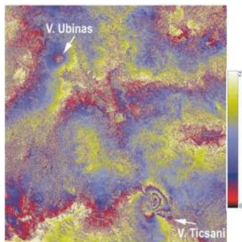
Figura 11. Interferograma obtenido para los volcanes Ubinas y Ticsani. La disposición de las franjas de color rojo y azul evidencia la existencia de deformación en la zona del volcán Ticsani. En el volcán Ubinas no se observa deformación (González et al., 2006).
