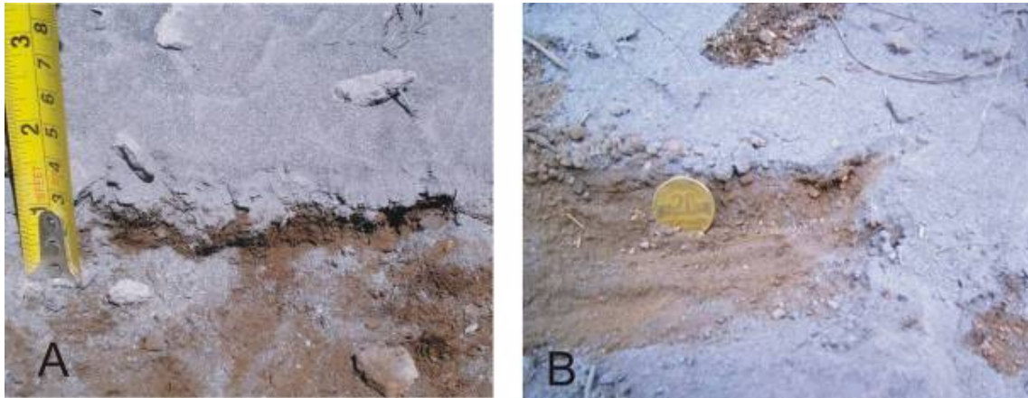
Figura 2. Depósitos de caída de ceniza: A) posee 1.5 cm de espesor aproximadamente a 3.5 km al SE del cráter del volcán Ubinas; B) 0.4 cm a 9 km al SE del cráter.
