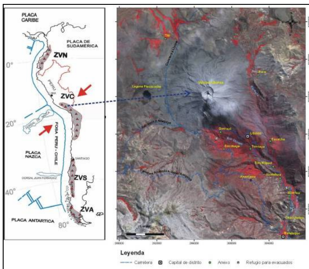
Figura 1. Distribución de las zonas volcánicas activas de Sudamérica (izquierda) e imagen de satélite que muestra al volcán Ubinas y las localidades aledañas.
