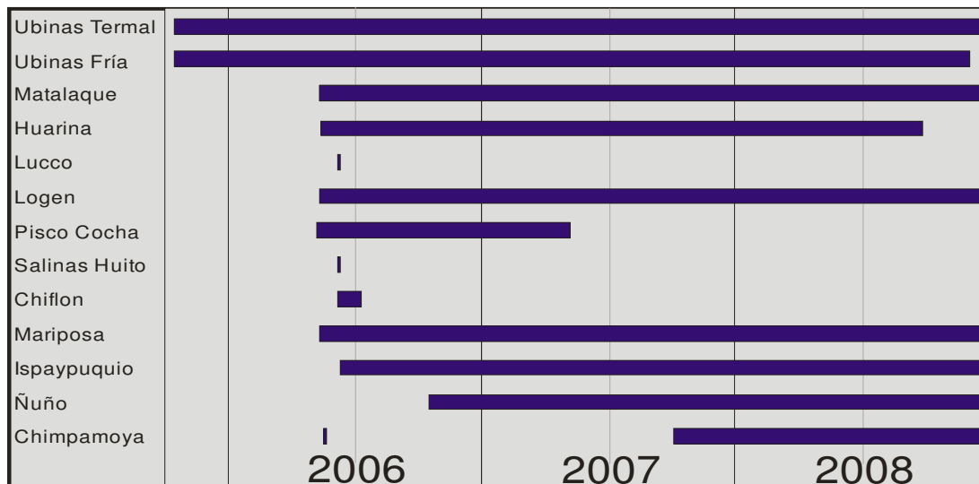
Figura 5. Periodos de monitoreo de las fuentes de aguas termales y frías, ubicadas alrededor del volcán Ubinas.
