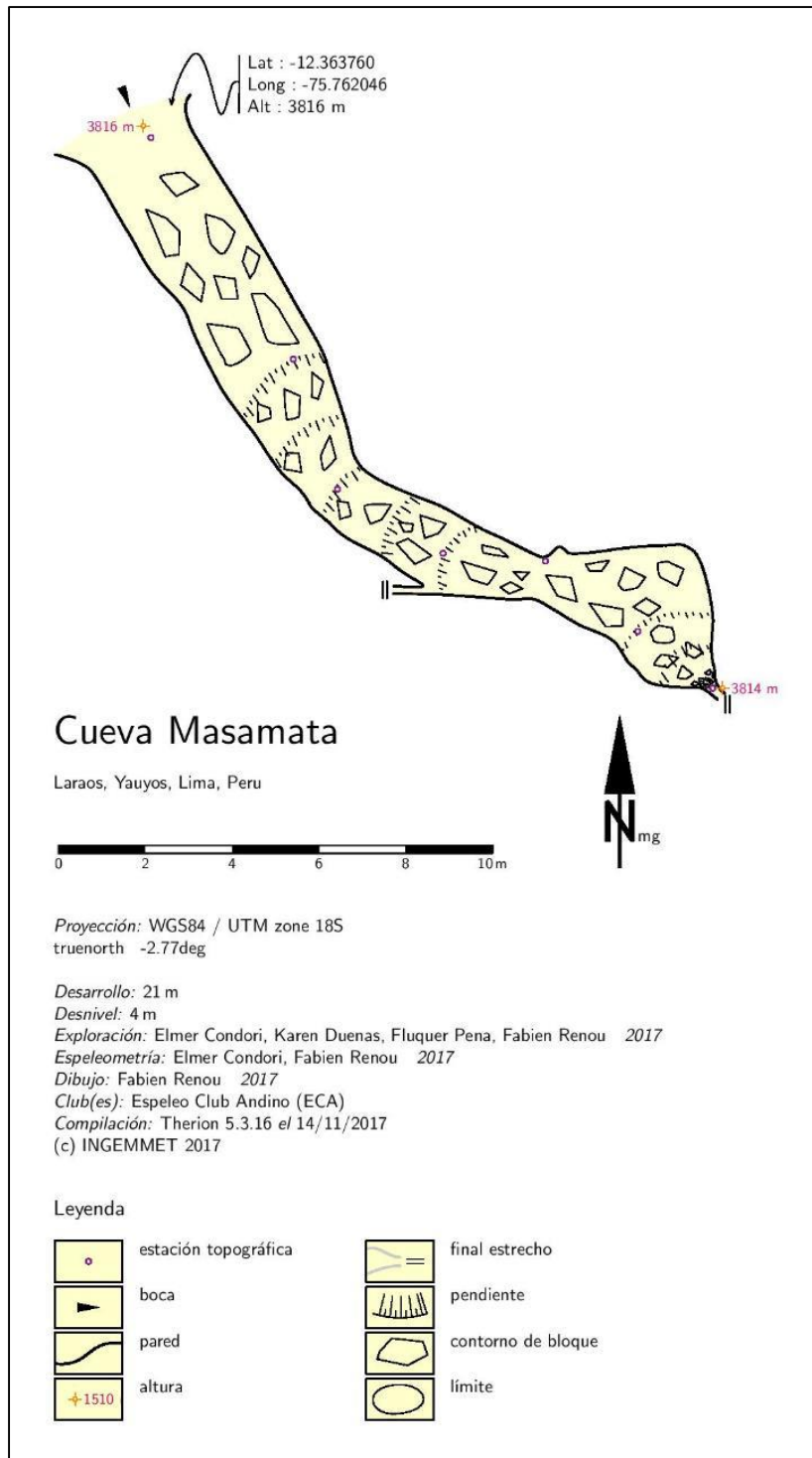
Figura 1: mapa de la cueva de Masamata
