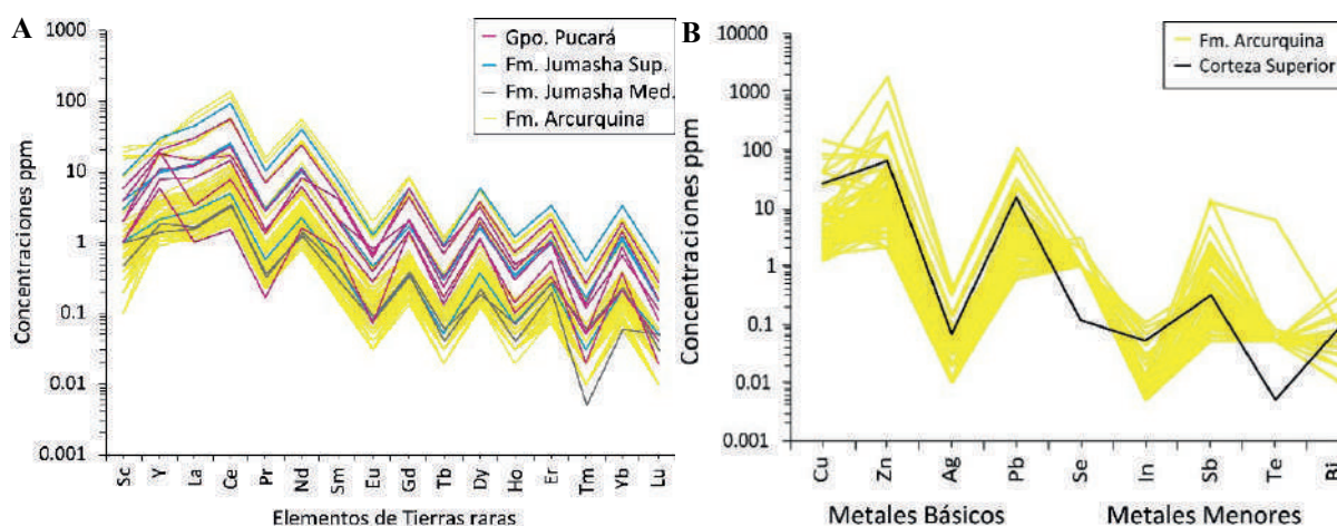
Figura 3: A. Perfil de concentración de las REE ordenadas por el número atómico vs la concentración en ppm, del Grupo Pucara, Formación Jumasha (medio y superior) y de la Formación Arcurquina. B. Perfil de concentraciones de los metales base de la Formación Arcurquina y de la Corteza Continental.
