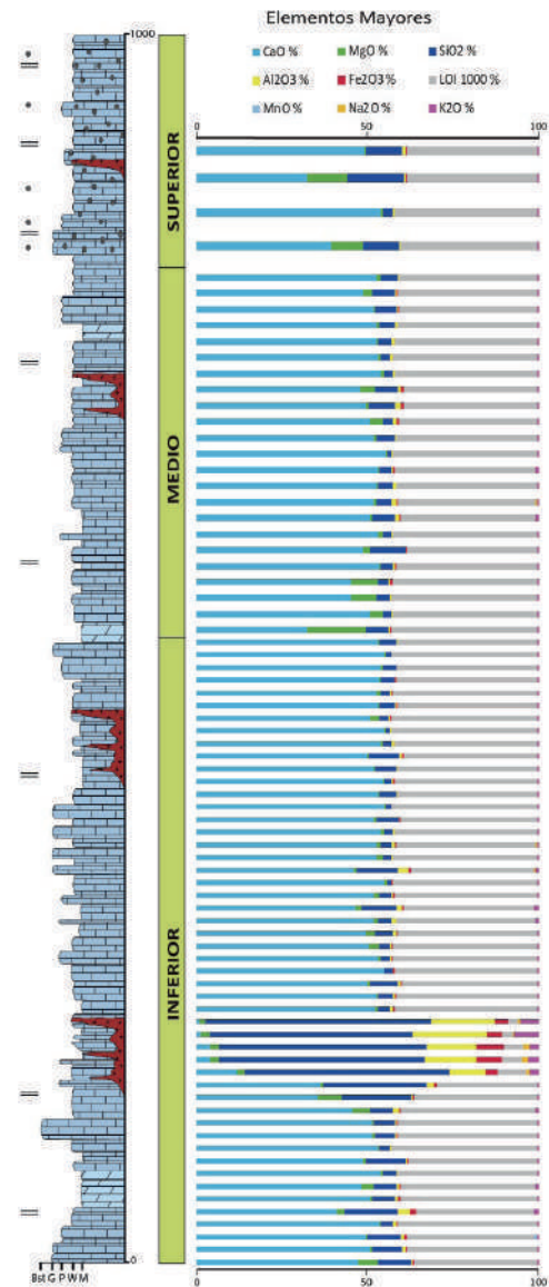
Figura 2: Columna integrada de la Formación Arcurquina caracterizada en base a su contenido químico de elementos mayores.
