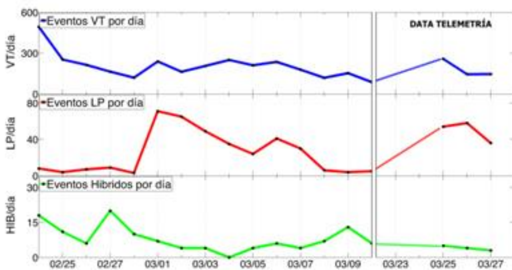
Figura 3: Gráfico estadístico de la sismicidad en la zona del volcán Sabancaya
