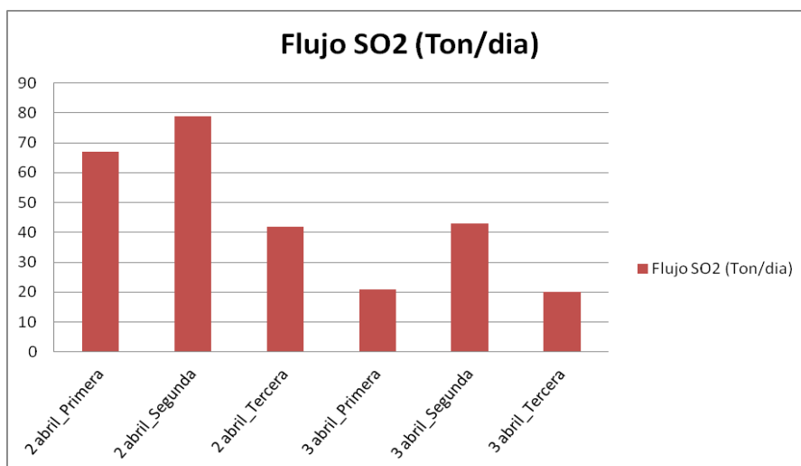
Figura 5: Valores de flujo de SO 2 medidos con espectrómetro mini-DOAS, los días 02 y 03 de Abril 2013
