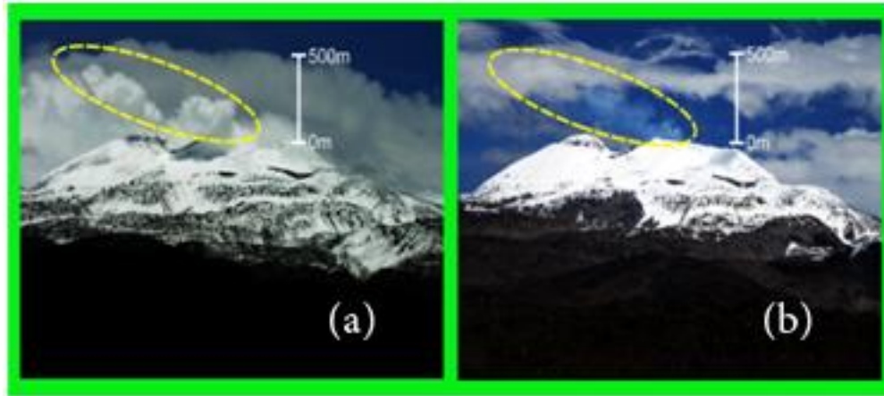
Figura 6: Fotos de la actividad fumarólica. En (a) se observa fumarolas blanquecinas y grises, que ocurren con mayor frecuencia, mientras que en (b) se observa emisiones azulinas, las cuales comenzaron a observarse el 14 de marzo, y que desde entonces han sido observados en diversas oportunidades..
