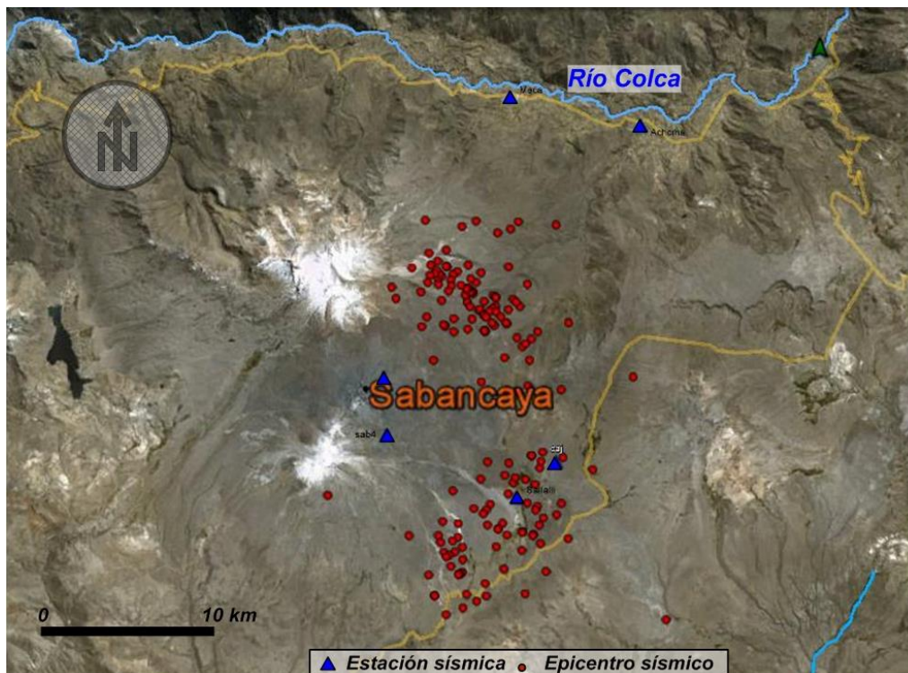
Figura 4: Mapa de la sismicidad observada entre el 23/02/2013 y el 17/03/2013. Los triángulos azules corresponden a la posición de las estaciones sísmicas
