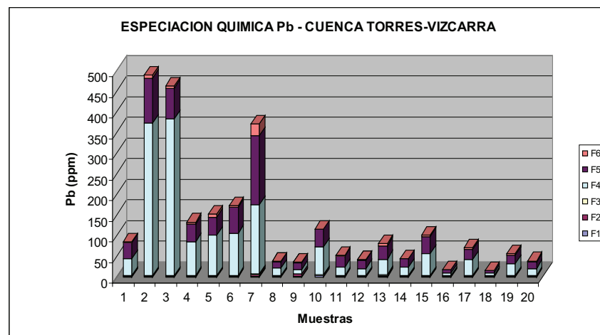
Fig. 1. Especiación química del plomo.
