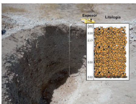
Fig. 5 – Sección geológica en Chimpapampa, donde se puede apreciar las 4 capas de pómez de la caída pliniana, 1) lapilli de pómez con abundantes líticos, 2) pómez con manchas hidrotermalizadas, 3) pómez ligeramente alargadas, 4) nivel de ceniza fina.
