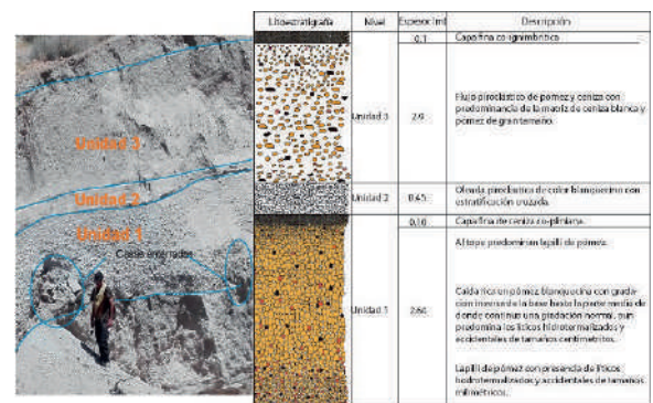
Fig. 2 - Columna estratigráfica de las 3 primeras unidades estratigráficas de los depósitos piroclásticos de la erupción del Huaynaputina 1600 d.C. en la Quebrada Calicanto.
