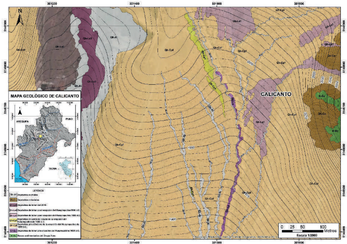
Fig. 1 – Mapa Geológico de la zona de Calicanto a escala 1/2000.
