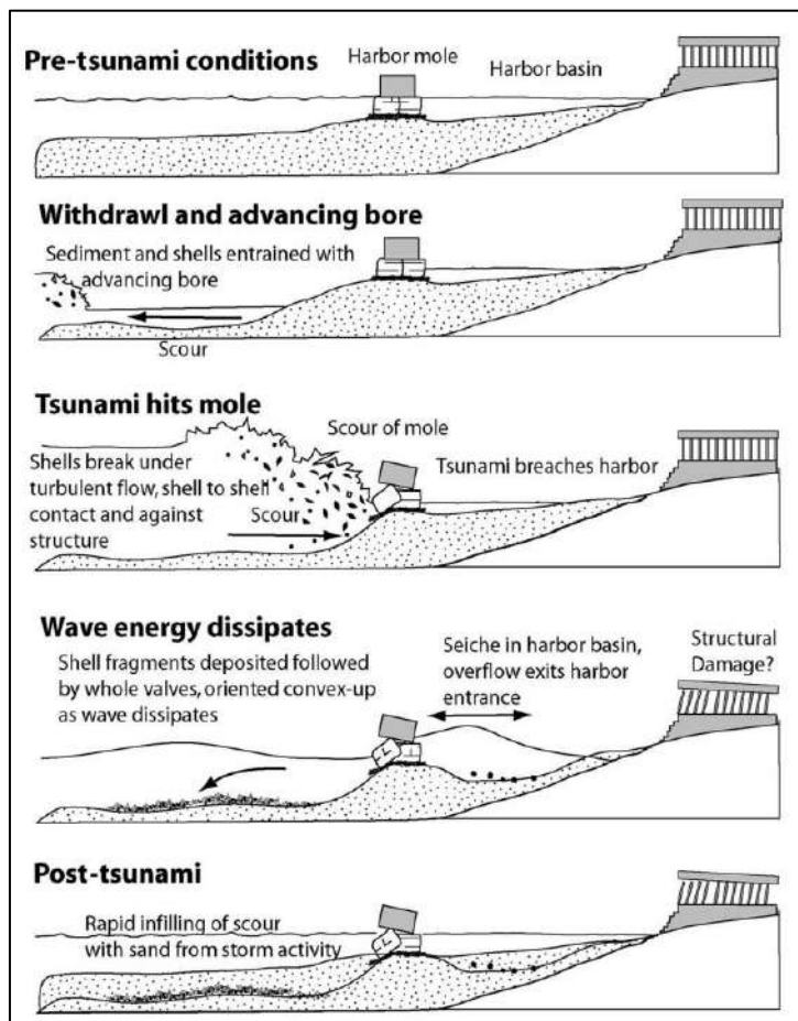
Fig. 3. Sequenza degli eventi causati da uno tsunami sul porto di Cesarea (da REINHARDT et alii 2006, fig. 4).
