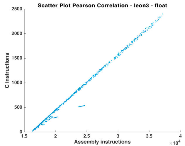
(d) LEON3 float Corr.
