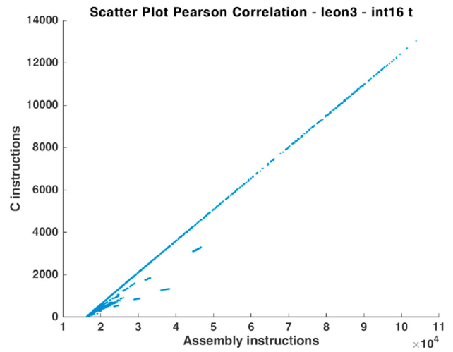
(b) LEON3 int16 Corr.
