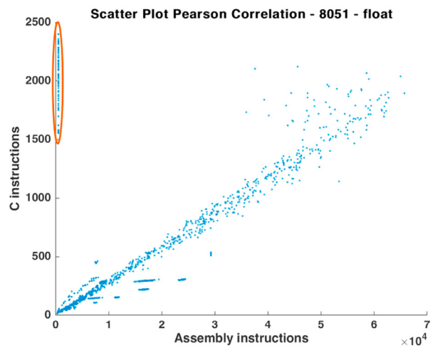
(d) 8051 float Corr.
