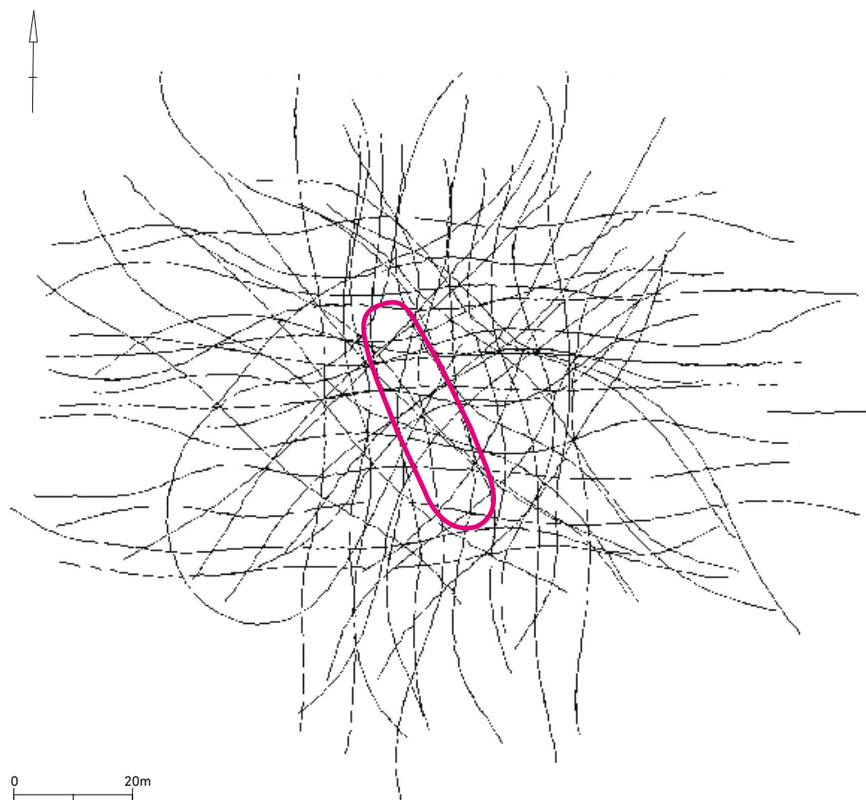
FIG. 10 Seismic network recorded over the wreck site of 't Vliegent Hart in 2010. The red ellipse marks the (supposed) location of the wreck. In total 49 profiles were recorded crossing the wreck at different angles. Seismisch netwerk opgenomen over het wrak van 't Vliegent Hart in 2010. De rode ellips markeert de (vermeende) locatie van het wrak. In totaal werden 49 profielen opgenomen die het wrak kruisen onder verschillende hoeken.
