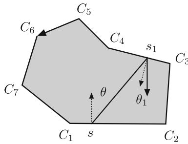
Fig. 1. Billiard map \Phi_f
