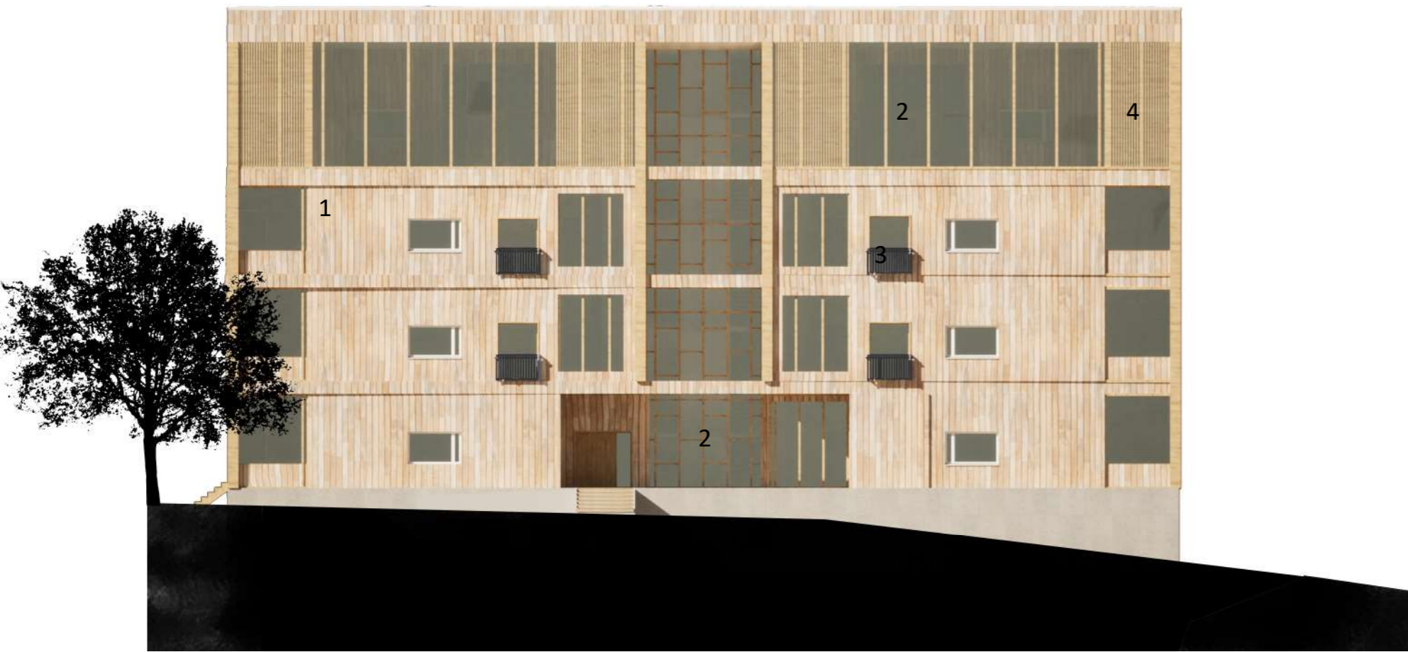
JULKISIVU LUOTEeseen
