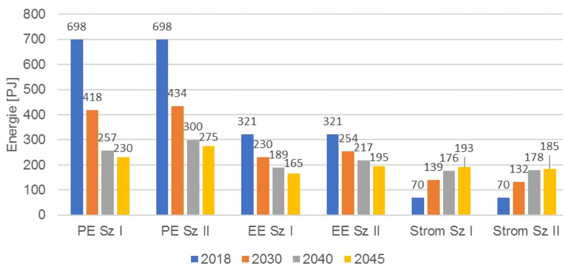
Abbildung 12: Szenarienvergleich – Primärenergie, Endenergie und Stromverbrauch 2030, 2040 und 2045 im Vergleich mit bisheriger Entwicklung (2018)
