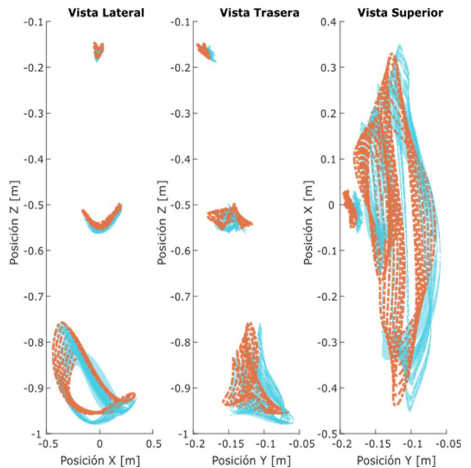
Figura 4. Visualización de las trayectorias de un sujeto (N19) a sus 8 velocidades de marcha. Las trayectorias reales medidas en azul y las reconstruidas en naranja. Como se puede apreciar la estimación de eventos cinemáticos y posterior reconstrucción se ajusta a las medidas reales se adecua a las trayectorias reales.
