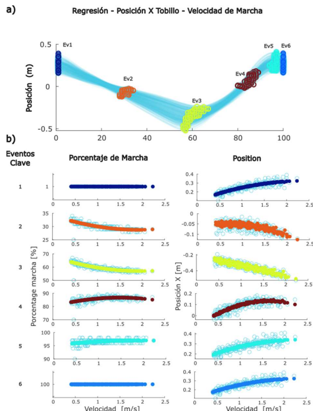
Figura 3. Esta figura proporciona una comparación entre los datos analizados y modelados de las trayectorias en el eje X del tobillo de todos los participantes en la base de datos. a) Trayectorias medidas en el durante la marcha del tobillo en el eje X junto a sus 6 eventos cinemáticos clave. b) Estimaciones mediante regresiones multivariable robustas de los eventos clave medidos (posición en el espacio y fase de la marcha) para cada participante en la base de datos.
