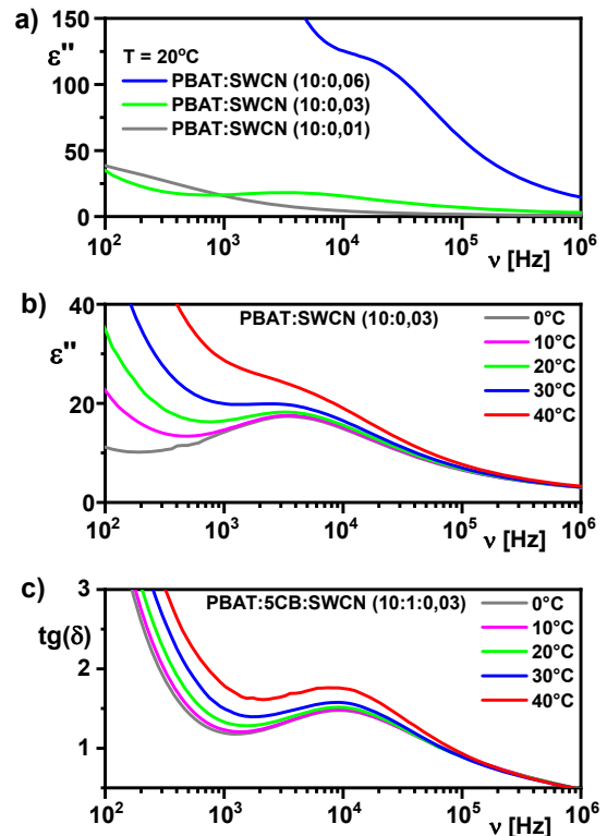
Rys. 3. Wpływ stężenia nanorurek węglowych na absorpcję dielektryczną PBAT:SWCN (a) oraz wpływ temperatury na relaksację przewodnictwa nanorurek węglowych w materiale dwuskładnikowym PBAT:SWCN (10:0,03) (b) i trójskładnikowym PBAT:5CB:SWCN (10:1:0,03) (c)
