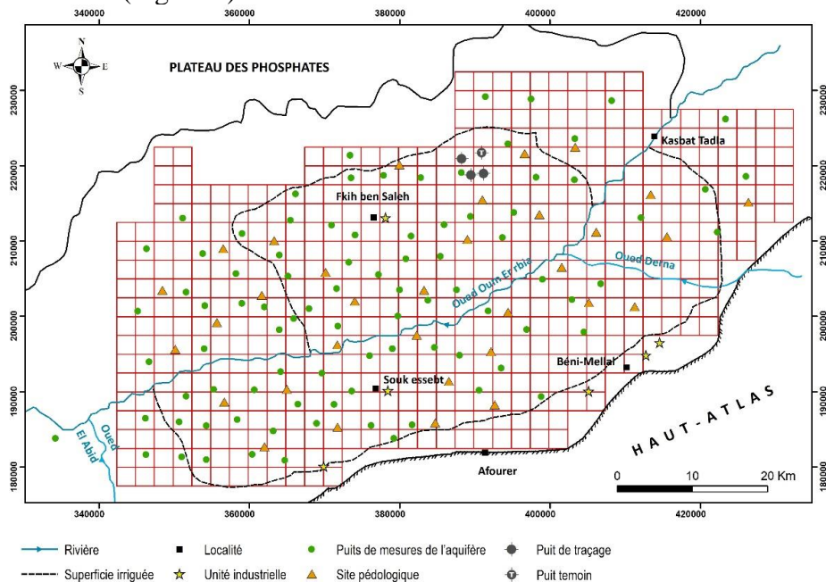
Figure 3. Carte schématique du bassin du Tadla et maillage de l'aquifère mio-plio-quaternaire
