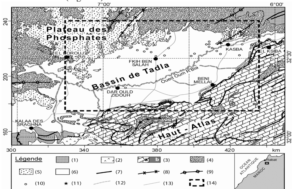
Figure 1. Carte géologique du bassin de Tadla. (1) Paléozoïque (schistes et quartzites). (2) Trias (argiles rouges et basalte). (3) Jurassique (a, calcaires et dolomies, b, diorite et gabbro). (4) Crétacé (faciès détritique rouge). (5) Tertiaire (calcaires, marnes et sables phosphatés). (6) Quaternaire (alluvions). (7) Faille. (8) Axe synclinal. (9) Axe anticlinal. (10) Forage. (11) Ville. (12) Rivière. (13) Route.
