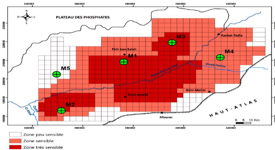
Figure 11. Carte de sensibilité à la pollution de l'aquifère mio-plio-quaternaire du bassin du Tadla. 1. Zone peu sensible, 2. Zone sensible, 3. Zone très sensible./avec les points de validation
