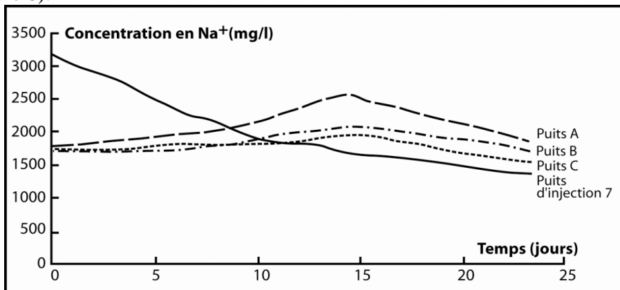
Figure 8. Evolution de la concentration en sel dans certains puits témoins
