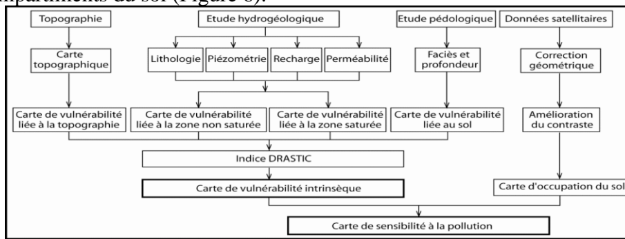
Figure 6. Organigramme d'élaboration de la carte de vulnérabilité intrinsèque des eaux souterraines par la méthode DRASTIC (Aller et al., 1987) .
