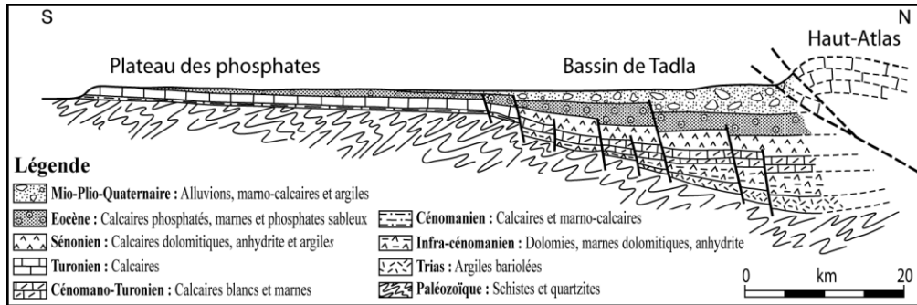
Figure 2. Coupe géologique montrant la structure du système aquifère du bassin de Tadla
