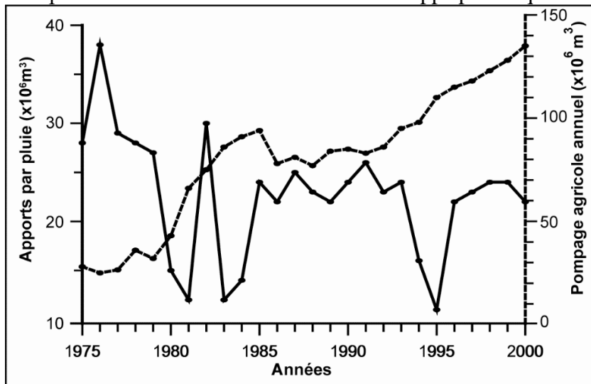
Figure 4. Evolution des apports de pluie dans le périmètre de Béni-Amir (en millions de \text{m}^3 ) et Evolution annuelle du pompage agricole à partir de la nappe de Béni-Amir (en millions de \text{m}^3 ).
