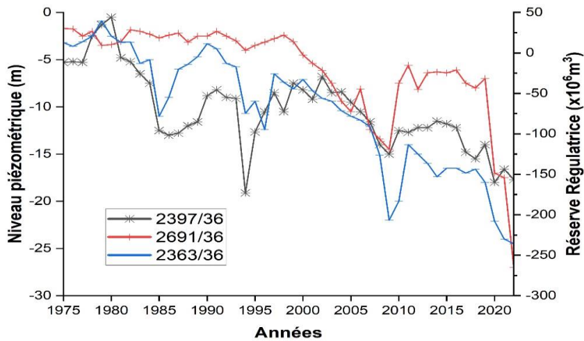
Figure 5. Evolution du niveau piézométrique (en mètres) dans les puits 2363/36, 2691/36 et 2397/36 de la plaine de Tadla et évolution de la réserve régulatrice de la nappe de Béni-Amir (en millions de m 3 )
