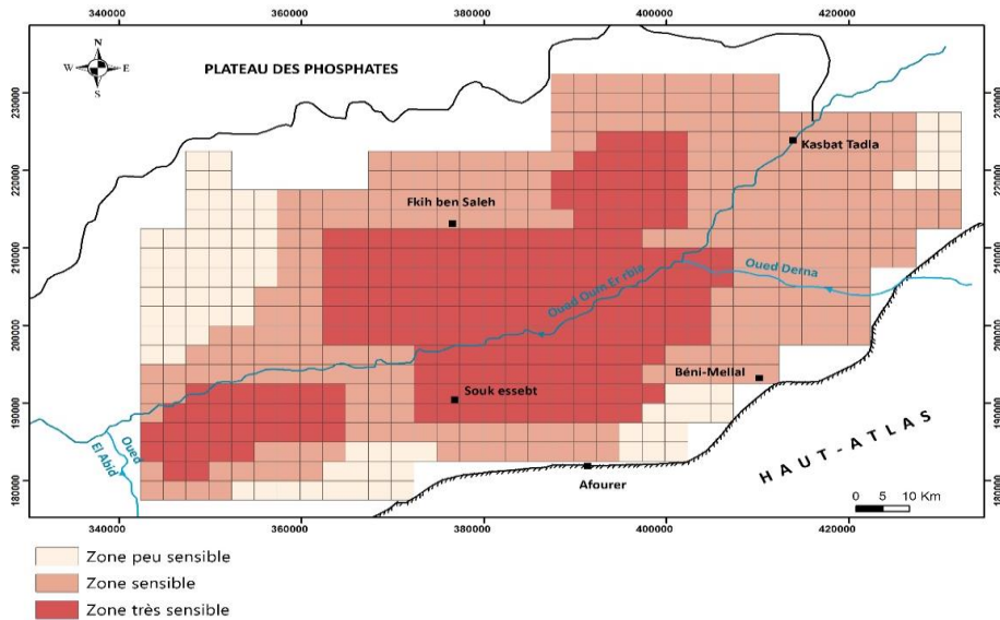
Figure 10. Carte de sensibilité à la pollution de l'aquifère mio-plio-quaternaire du bassin du Tadla. 1. Zone peu sensible, 2. Zone sensible, 3. Zone très sensible
