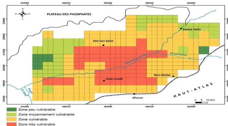
Figure 9. Carte de vulnérabilité intrinsèque à la pollution de l'aquifère mio-plio-quadernaire du bassin du Tadla. 1. Zone peu vulnérable, 2. Zone moyennement vulnérable, 3. Zone vulnérable, 4. Zone très vulnérable.
