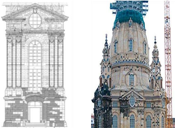
شكل 8 يوضح استخدام وإسقاط الأحجار القديمة مع الجديدة. المصدر: [31].
