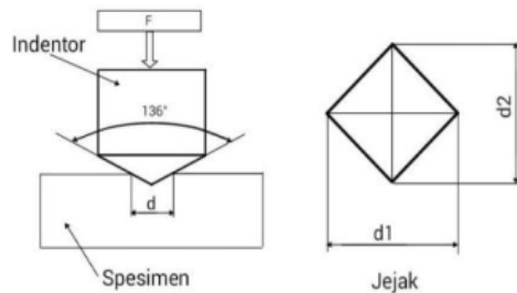
Gambar 2. Skema pengujian ekerasan vickers Sumber : (3)
