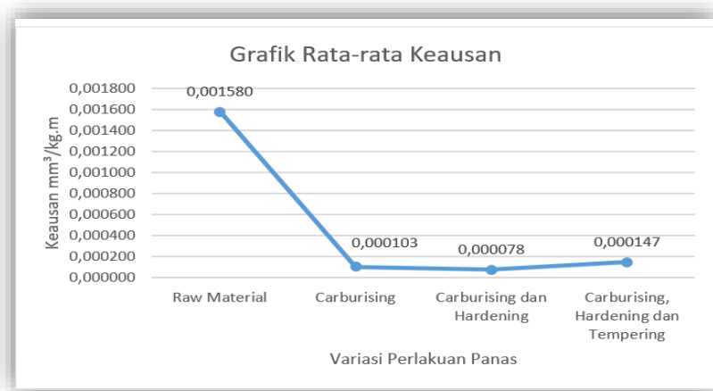
Gambar 6. Grafik Rata-Rata Keausan
