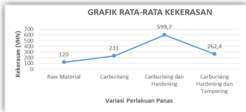
Gambar 5. Grafik Rata-Rata Kekerasan
