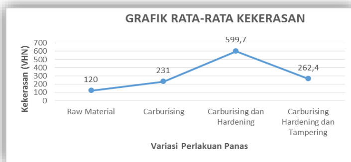
Gambar 5. Grafik Rata-Rata Kekerasan
