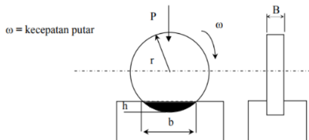
Gambar 3. Skema pengujian keausan metode Ogoshi
