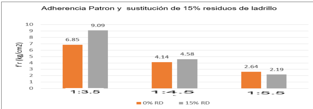
Fig. 27. Resistencia a la adherencia de elementos de albañilería.
