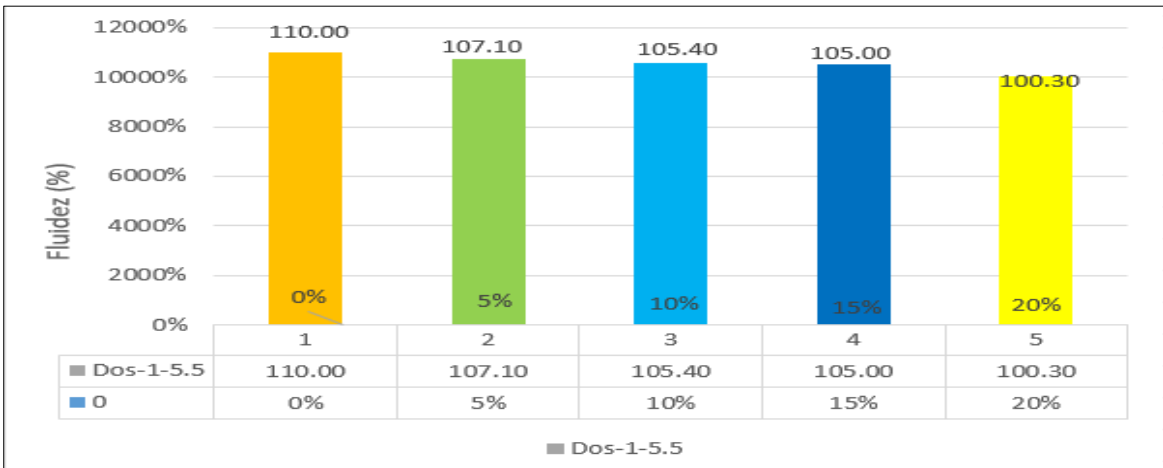
Fig. 15. Fuidez de mortero patrón y mortero con residuos de ladrillo en 1:5.5.
