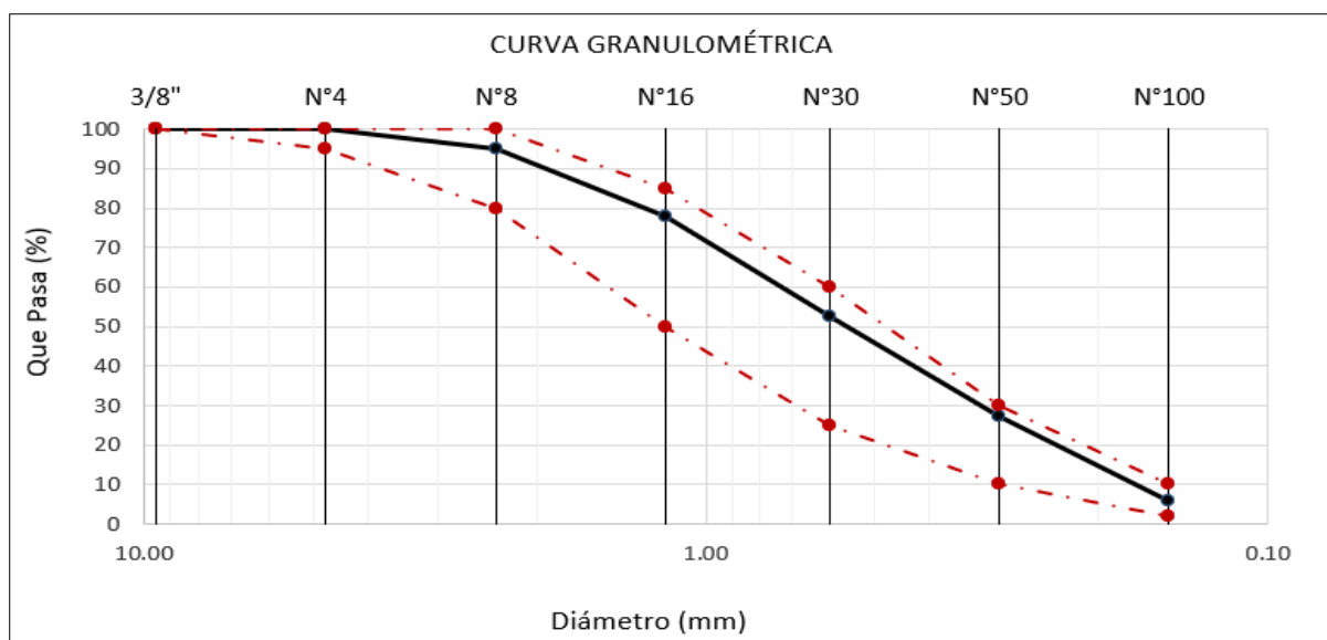
Fig. 9: Huso Granulométrico del Áridos, para Mortero: La victoria – Pátapo.
