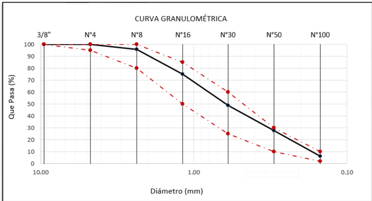
Fig. 10: Huso Granulométrico de los residuos de Ladrillo.
