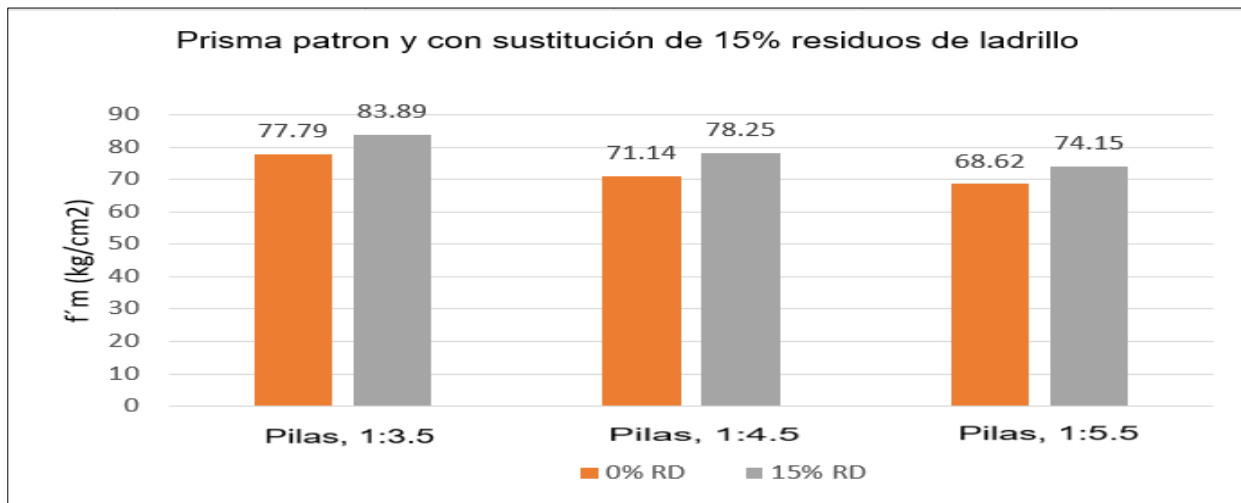
Fig. 25. Resistencia a la compresión de prismas de albañilería.
