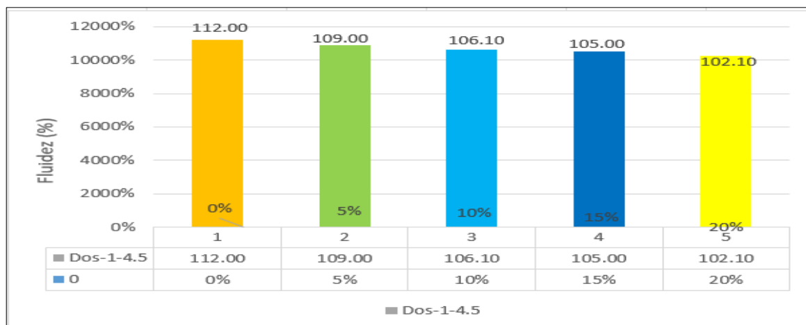
Fig. 14. Fluidez de mortero patrón y mortero con residuos de ladrillo en 1:4.5.
