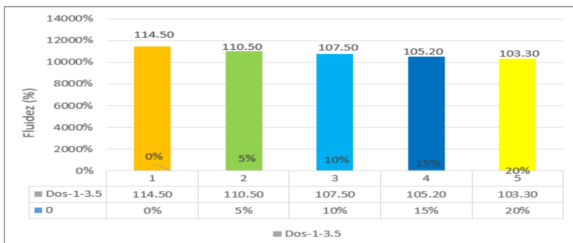
Fig. 13. Fluidez de mortero patrón y mortero con residuos de ladrillo en 1:3.5.
