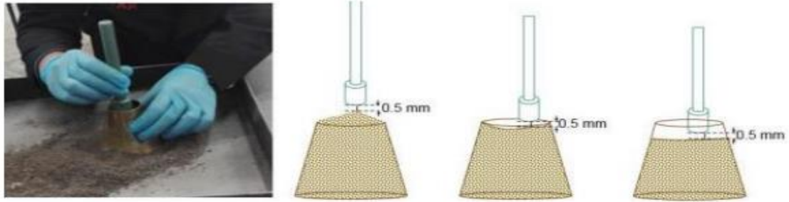
Fig. 7: Compactación del Árido, para verificar Condiciones [74].
