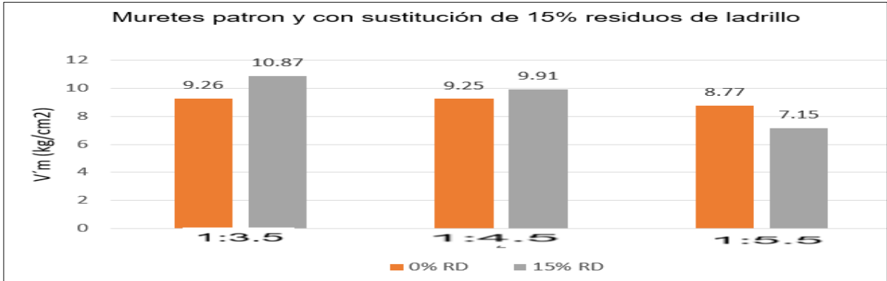
Fig. 26. Resistencia a la compresión diagonal de muretes de albañilería.
