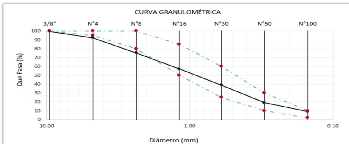
Fig. 11. Curva Granulométrica del Agregado: Tres Tomas Ferreñafe.
