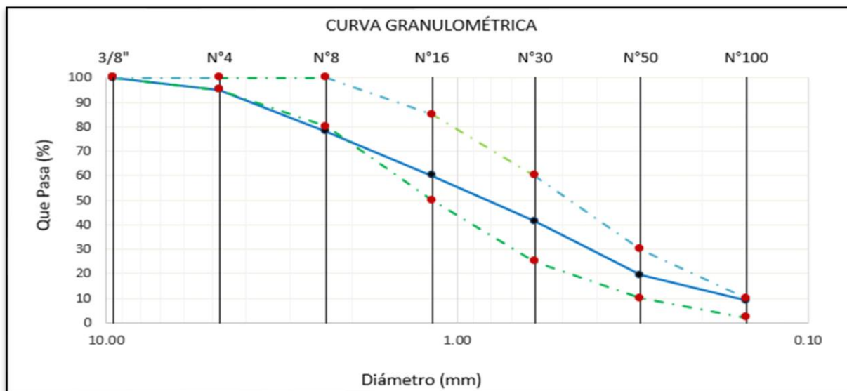
Fig. 12. Curva Granulométrica del Agregado: Pacherrez – Pucalá.
