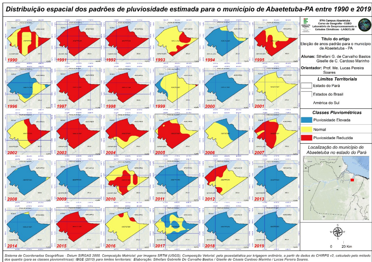
Figura 4 – Distribuição espacial dos padrões de pluviosidade estimada para o município de Abaetetuba-PA entre 1990 e 2019.
