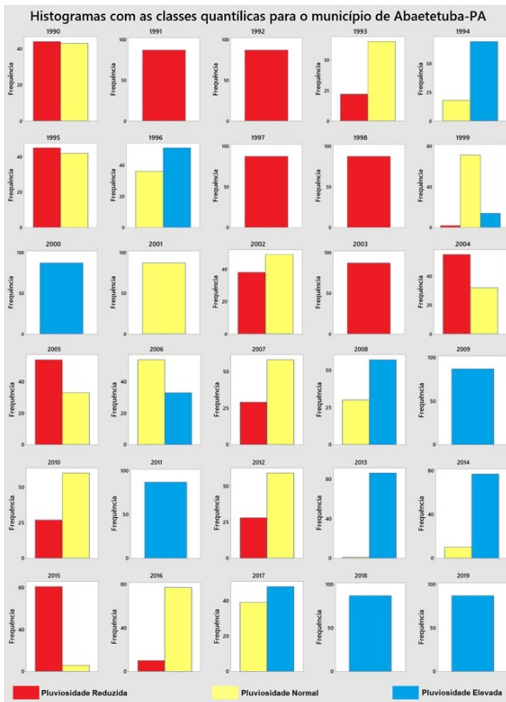
Figura 3 – Histogramas com as classes quantílicas para o município de Abaetetuba-PA.
