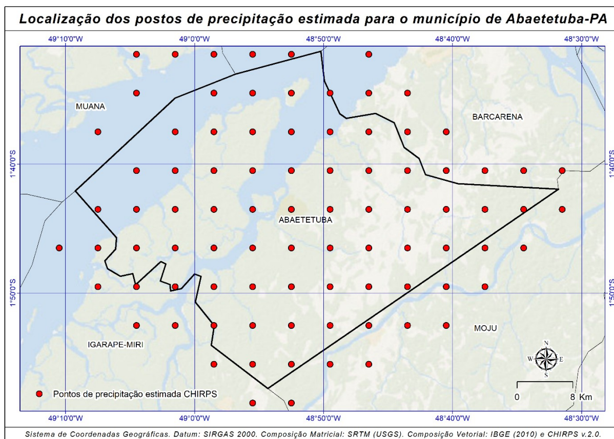
Figura 2 – Localização dos postos de precipitação estimada para o município de Abaetetuba-PA. Fonte: elaborado pelos autores.
