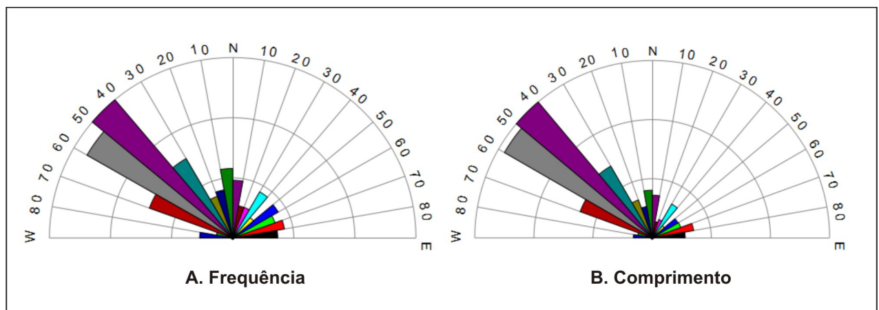
FIGURA 8. Diagrama de roseta dos Lineamentos Estruturais presentes na Carta Topográfica de Faxinal: A) direção preferencial de freqüência de Lineamentos N50°W. B) maior comprimento na mesma direção.
