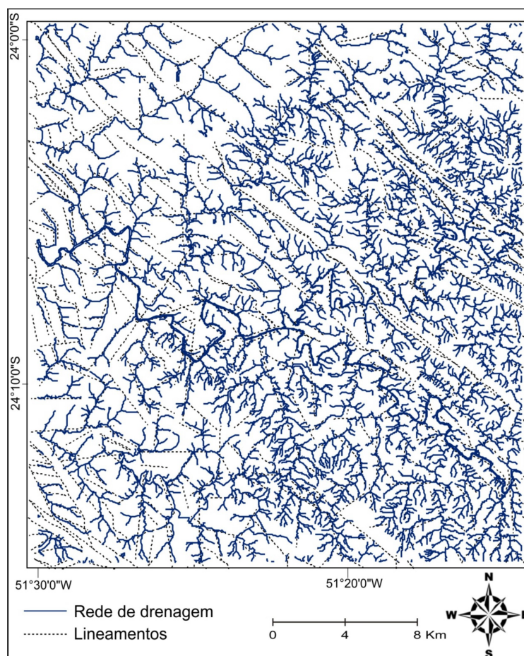
FIGURA 3. Configuração da rede de drenagem sobreposta a lineamentos estruturais extraídos do MDE da Carta de Faxinal.
