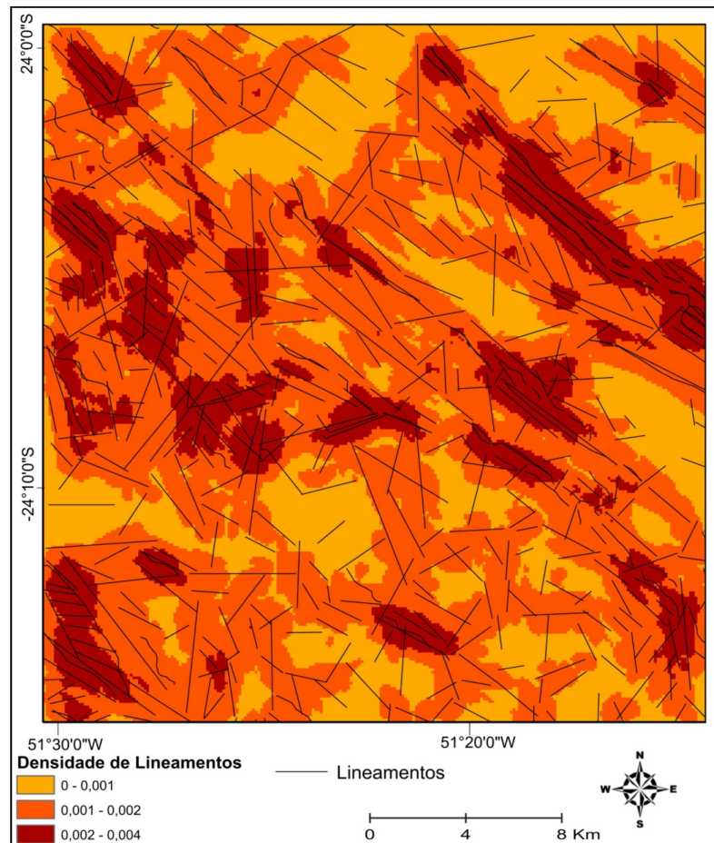
FIGURA 7. Mapa de densidade de Lineamentos da carta de Faxinal - PR, destacando maior densidade SE, W e extremo NE.
