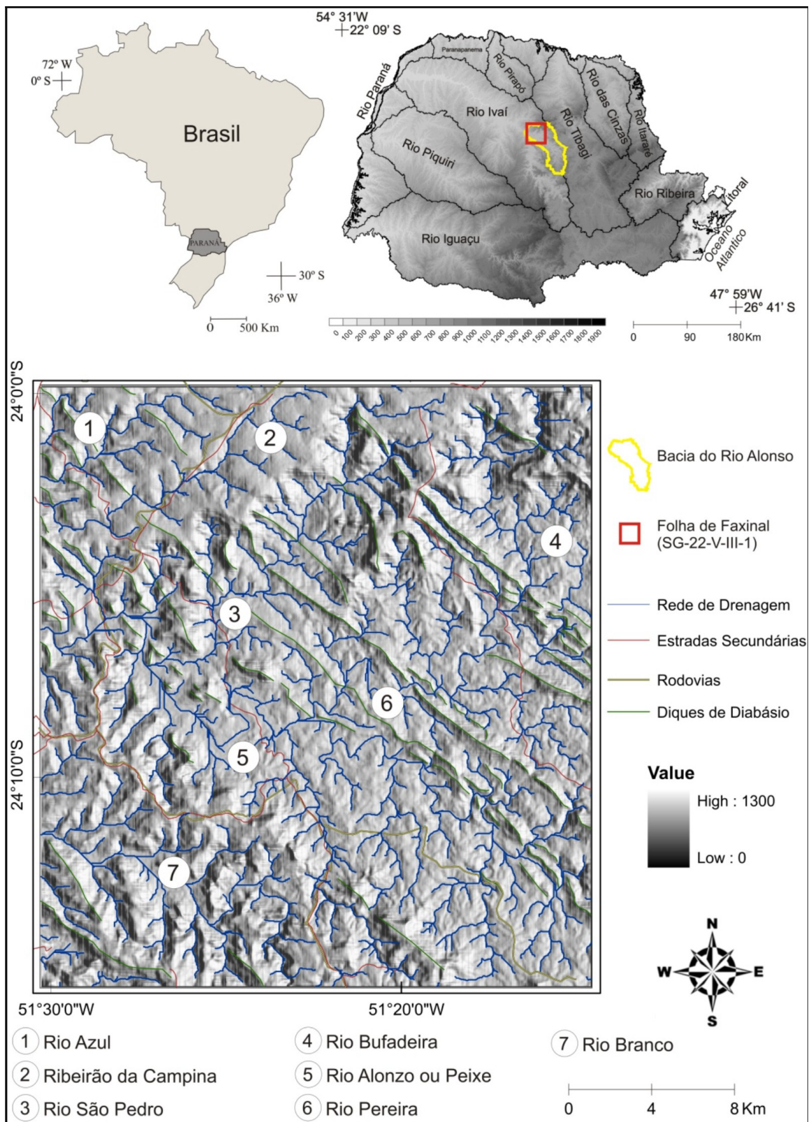
FIGURA 1. Mapa de Localização da área abrangida pela carta de Faxinal.
