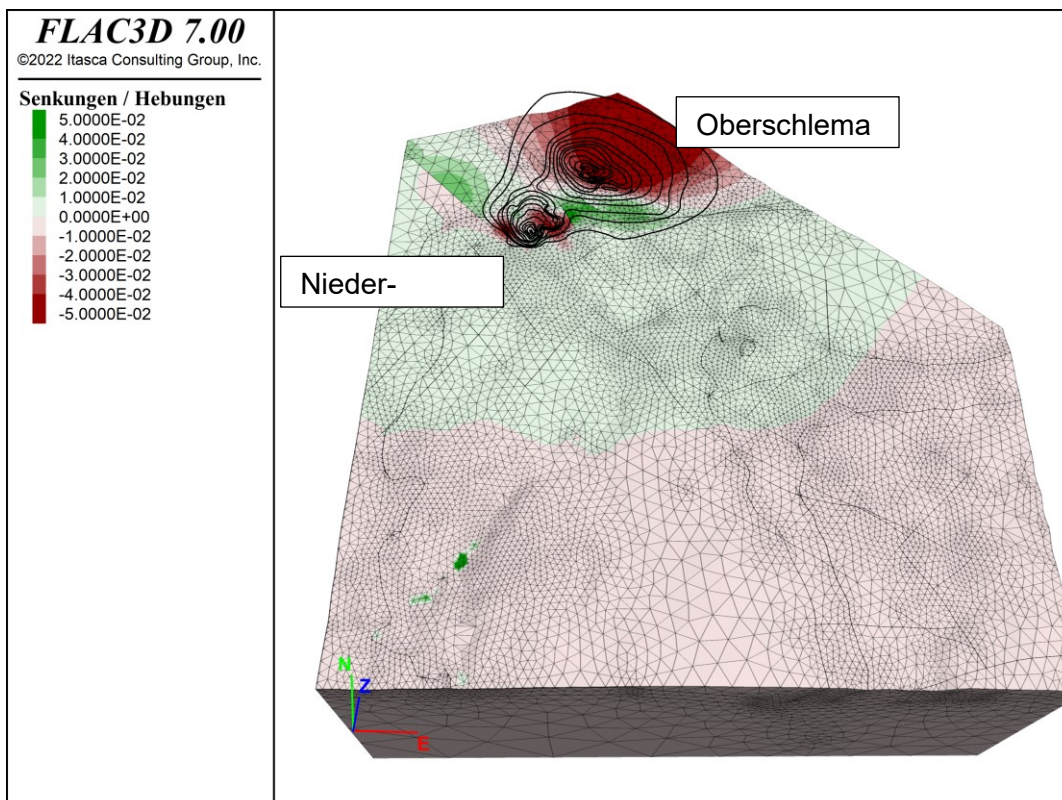
Abbildung 29: Modellierte Setzungen und Hebungen nach Grundwasserwiederanstieg. Die von der WISMUT GMBH (2020) ermittelten Senkungslinien sind als Referenz in der Abbildung dargestellt.
