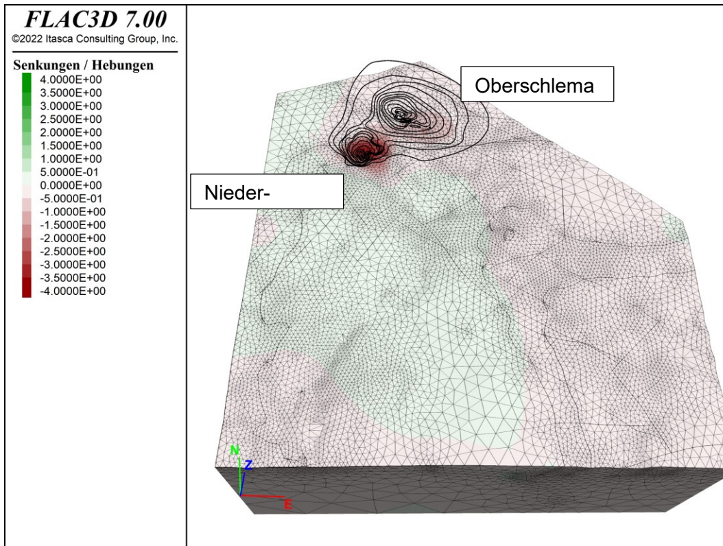
Abbildung 28: Modellierte Senkungen nach Ende der bergbaulichen Tätigkeit. Die von der WISMUT GMBH (2020) ermittelten Senkungslinien sind als Referenz in der Abbildung dargestellt.
