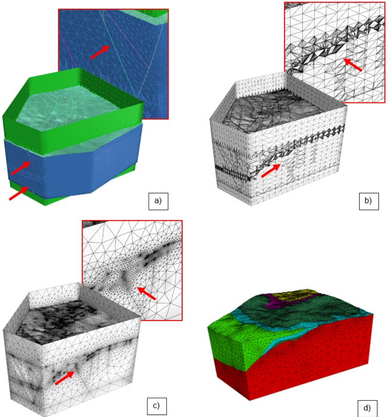
Abbildung 15: Bearbeitungsschritte in Rhinoceros zum Erzeugen eines Volumennetzmodells aus mehrfach bearbeiteten Oberflächennetzen: a) Die einzelnen Oberflächennetze wurden miteinander verschritten, sodass sie an der Schnittlinie gemeinsame Knotenpunkte (siehe rote Pfeile und Ausschnitt) besitzen. b) Die Teilnetze aus a) wurden in ein einziges Netz zusammengeführt. Überstehende Teilnetze wurden entfernt. c) Das Oberflächennetz wurde neu vernetzt, um die Zielauflösung des Volumennetzes anzupassen. (siehe rote Pfeile und Ausschnitt). Die Pfeile in b) und c) markieren jeweils die gleichen Modellbereiche. d) Volumennetzmodell in 3DEC: überstehende Oberflächennetze wurden automatisch entfernt.
