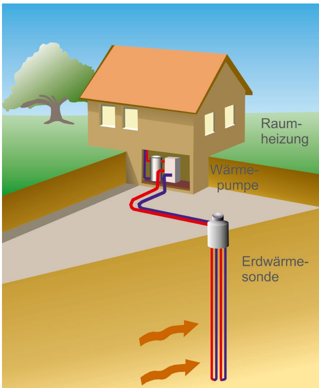
Abbildung 10: Schema Erdwärmesonde
