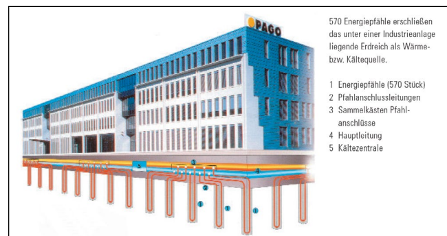
Abbildung 11: Schema erdberührte Betonbauteile
