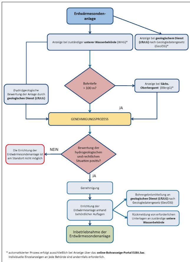
Abbildung 12: Schema Verfahrensablauf Genehmigungsprozess einer Erdwärmesondenanlage
