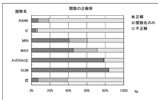
図9 関数の正解率
