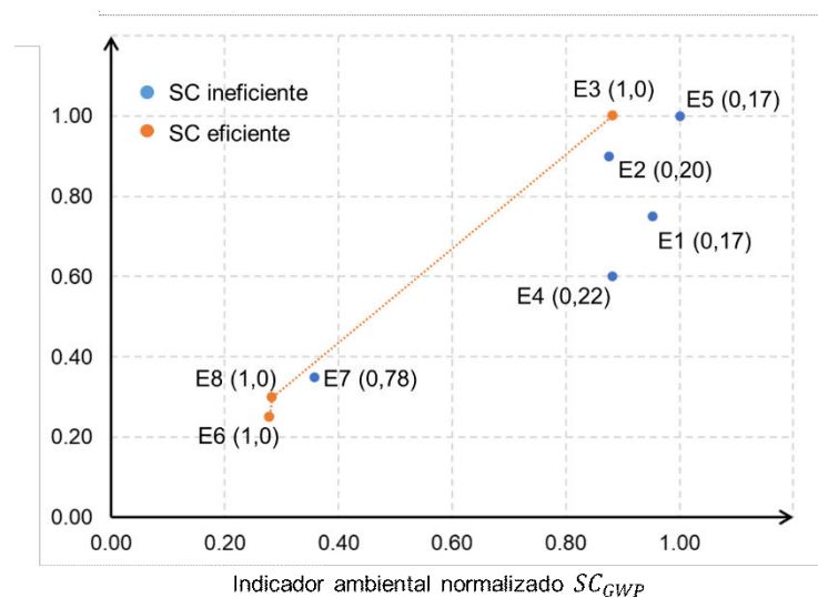
Fig. 4. Frontera de eficiencia. Los valores entre paréntesis son las eficiencias ( \rho ) para cada escenario E.
