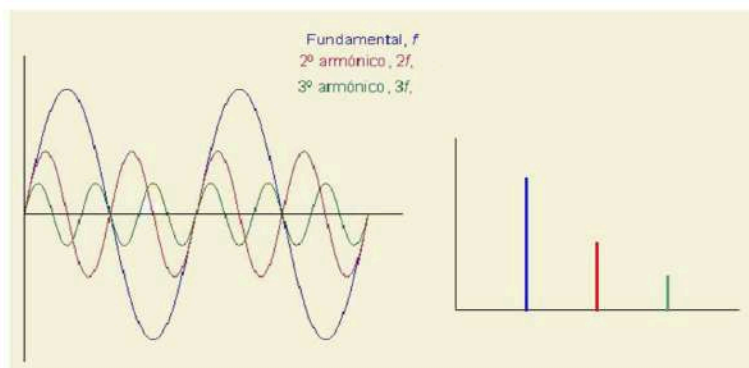
Figura 3.6: Primeros armónicos
