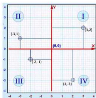
Figura 2.8: Puntos en el plano
