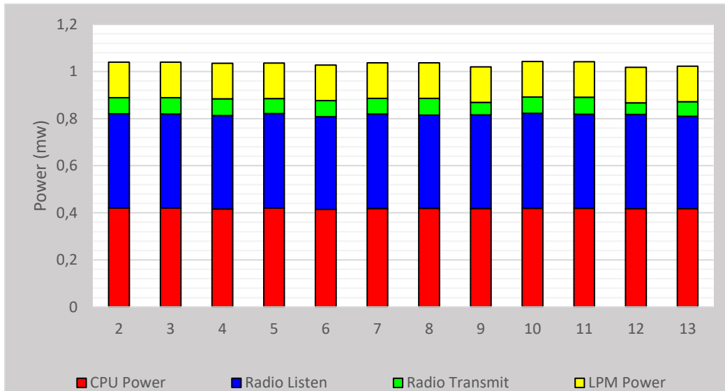
Histogramme 1 : Consommation moyenne d'énergie (architecture centralisée)
