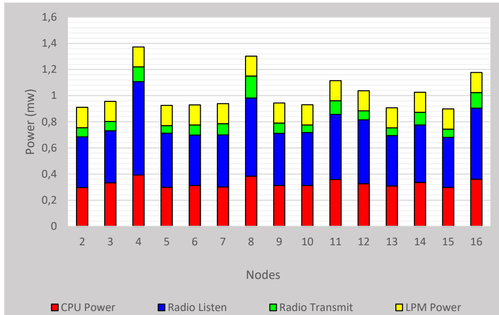
Histogramme 2 : Consommation moyenne d'énergie (architecture décentralisée)
