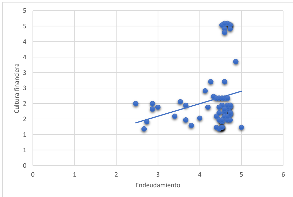
Gráfica de dispersión ( R^2 )
