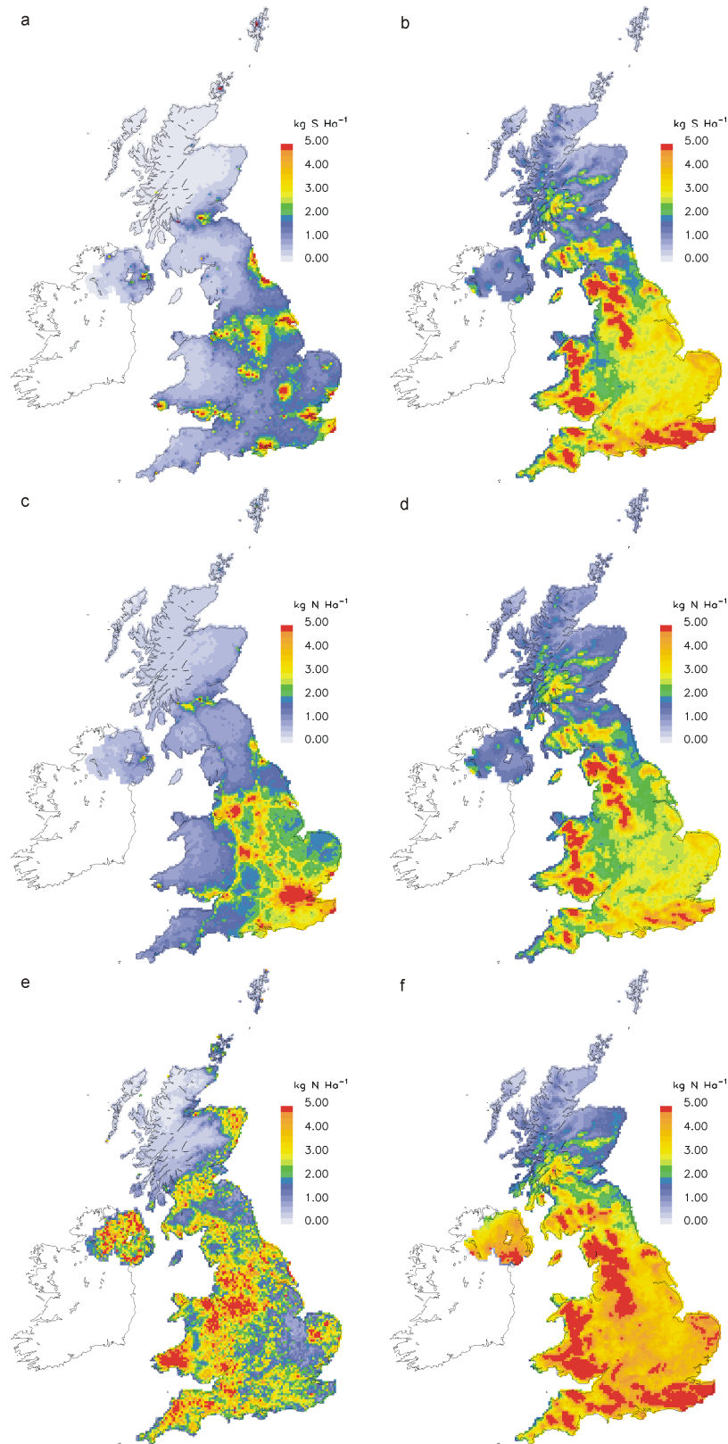
Fig. 9. FRAME 2020 deposition: a) SO x dry; b) SO x wet; c) NO y dry; d) NO y wet; e) NH x dry f) NH x wet (kg S or N ha -1 yr -1 )
