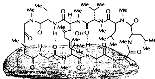
(a) CsA
