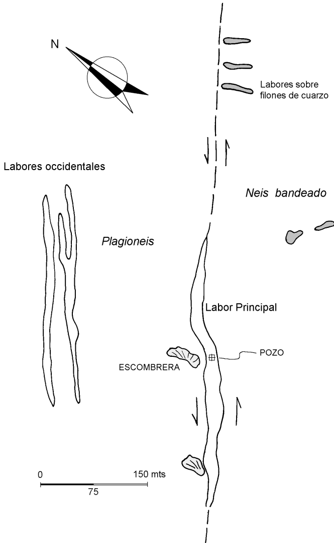
Fig. 3 -Fosas de Vila.- Esquema de las labores
