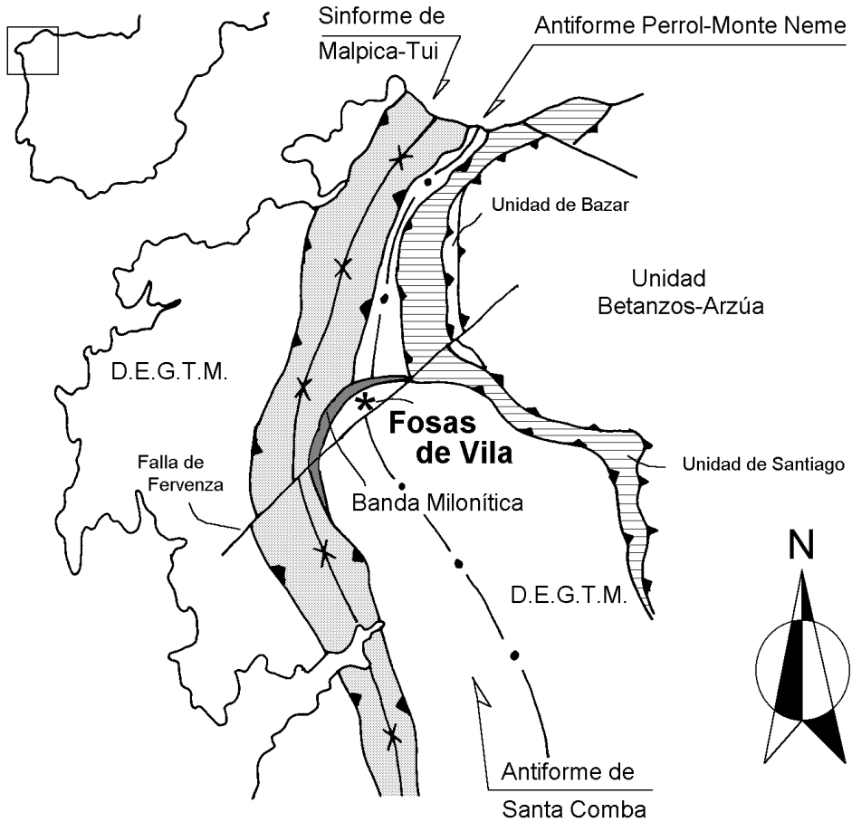
Fig. 1 -Situación del área de estudio. Modificado de IGME 1984
