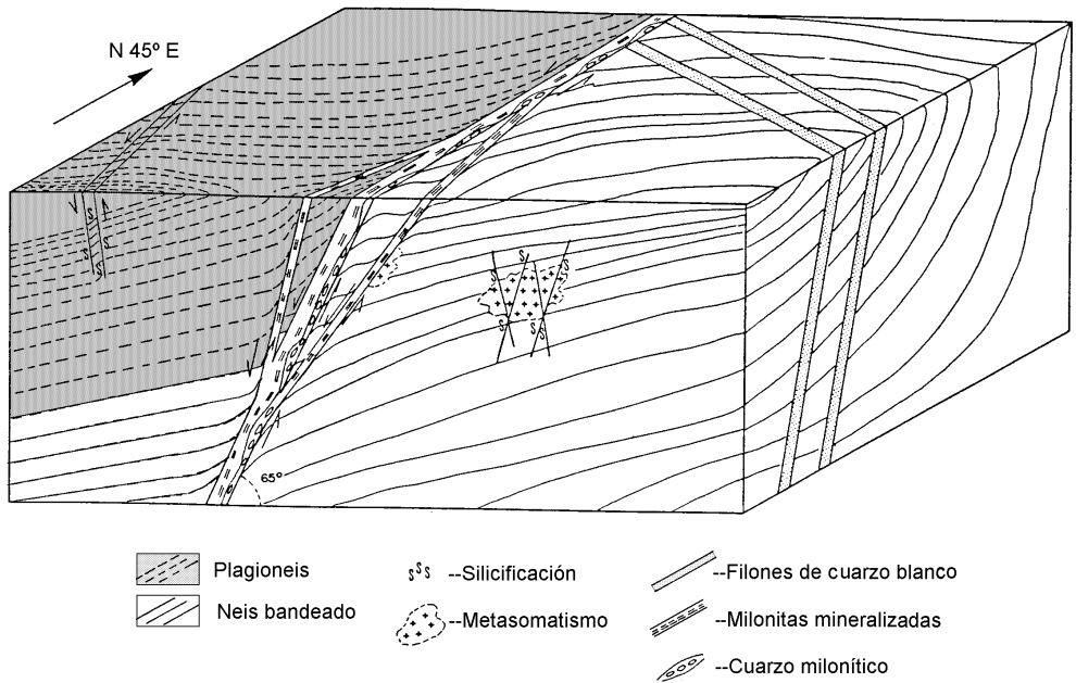
Fig. 4 - Fosas de Vila.- Bloque diagrama
