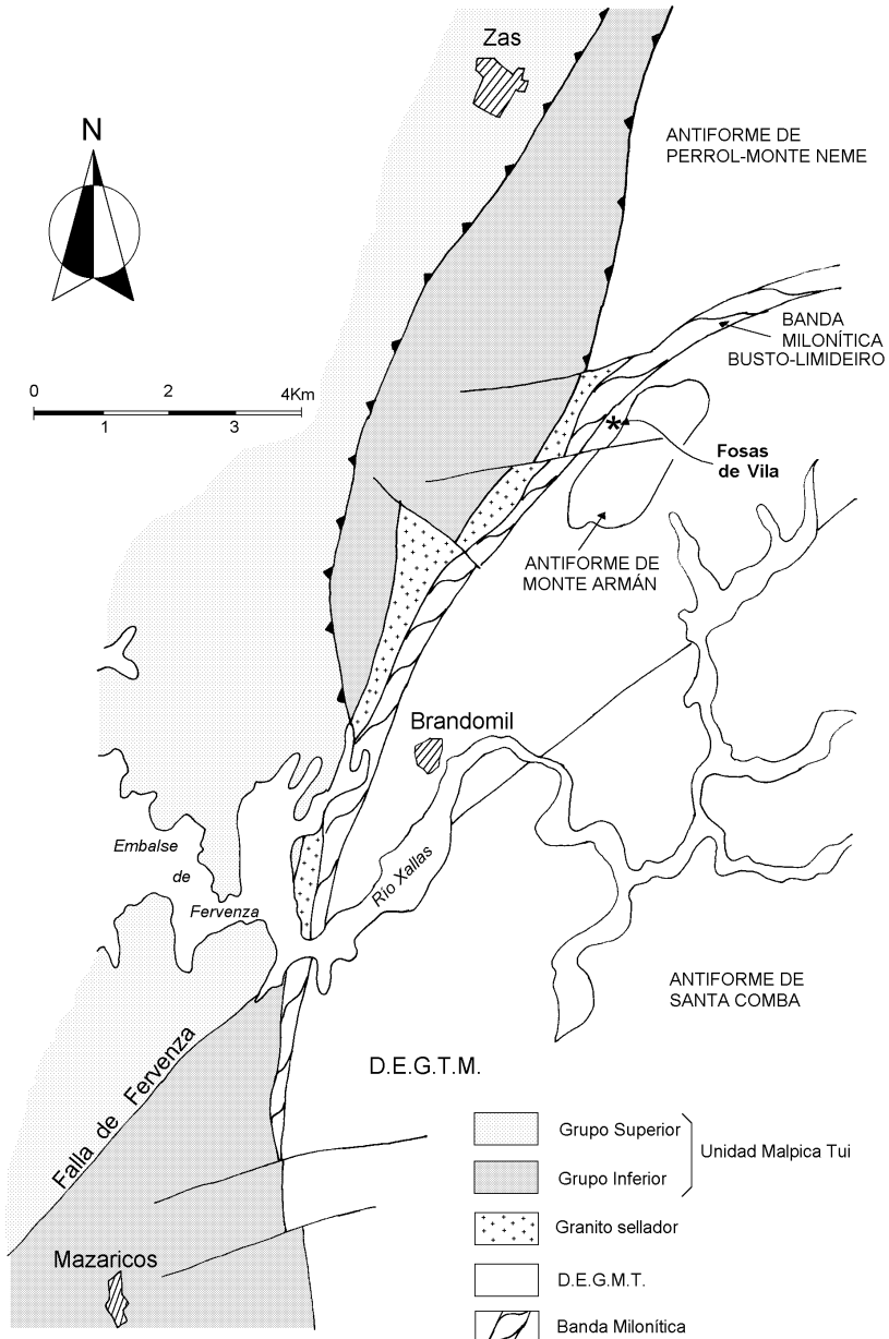
Fig. 2 -Configuración geológica del entorno de Fosas de Vila
