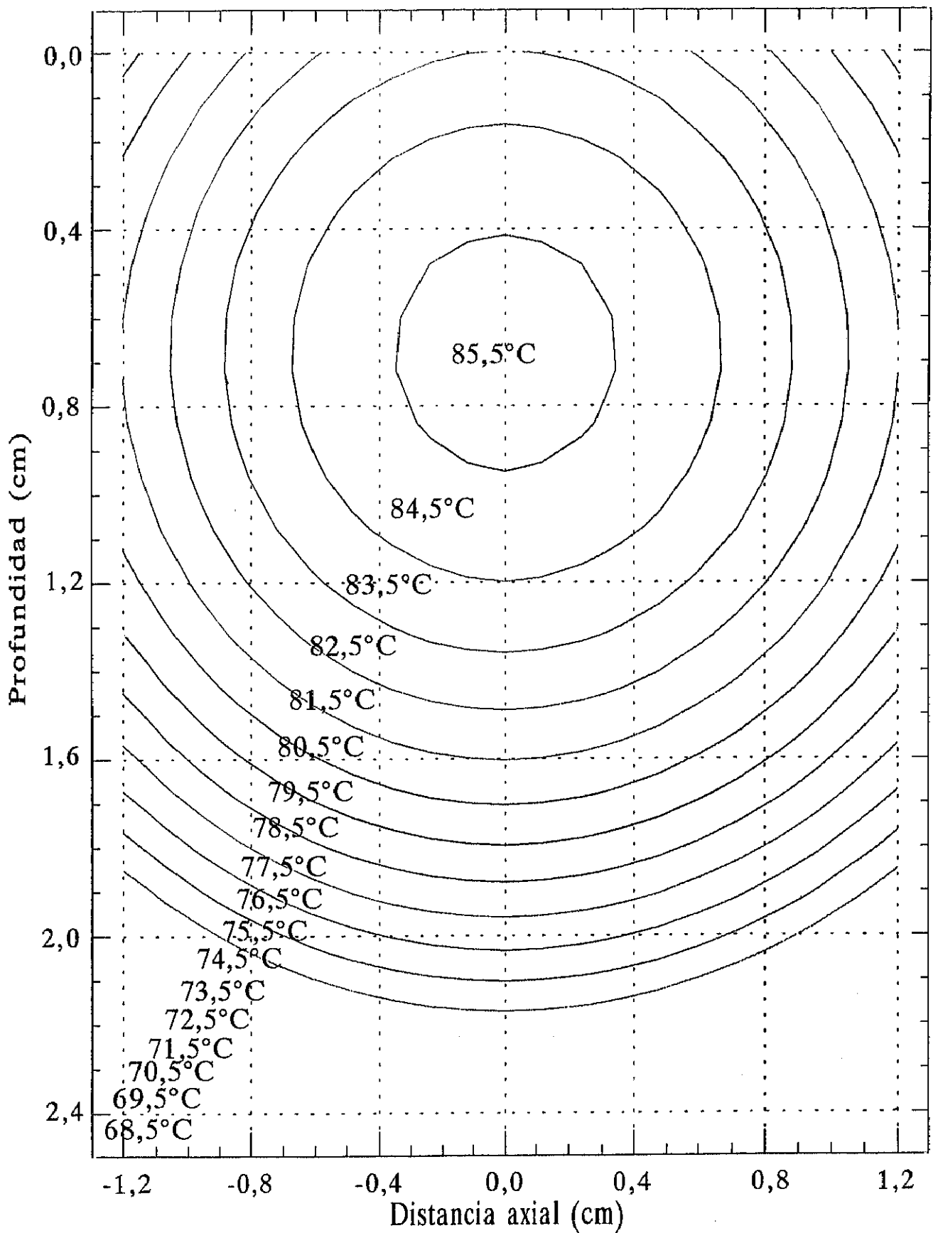
Figura 17. Curvas de nivel de la temperatura en función de la profundidad y la distancia axial, correspondientes al calentamiento de leche con microondas en discontinuo durante 30 segundos.
