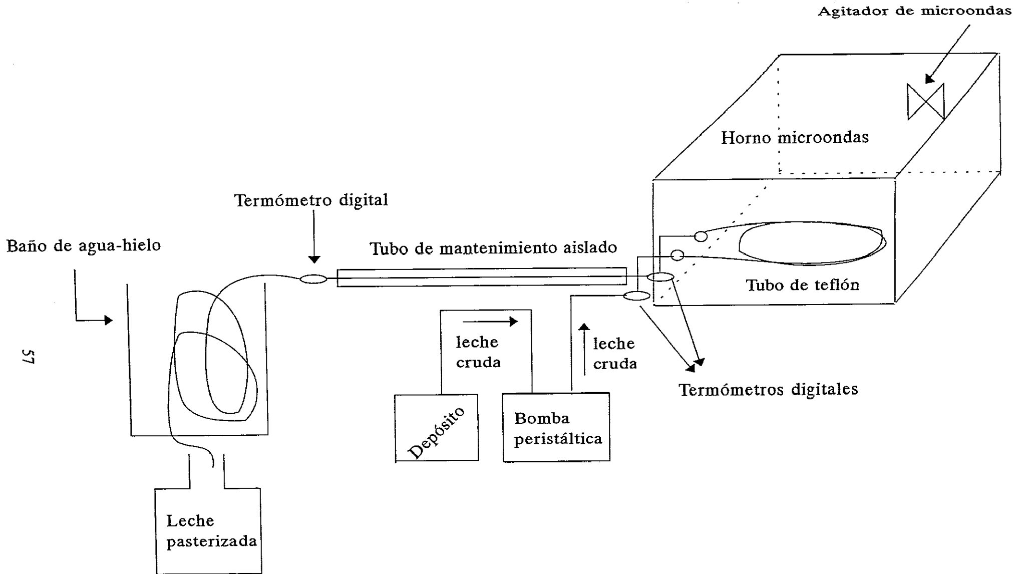
Figura 8. Esquema del sistema de pasteurización con microondas.
