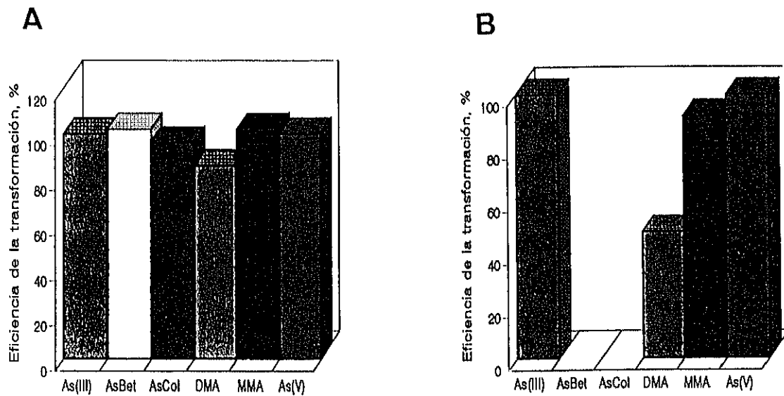
Figura 16.- Eficiencia en la generación de hidruros para As(III), As(V), MMA, DMA, AsB y AsC, (A) con termo-oxidación y (B) sin termo-oxidación. Concentración de As: 200 \mu\text{g L}^{-1} .
