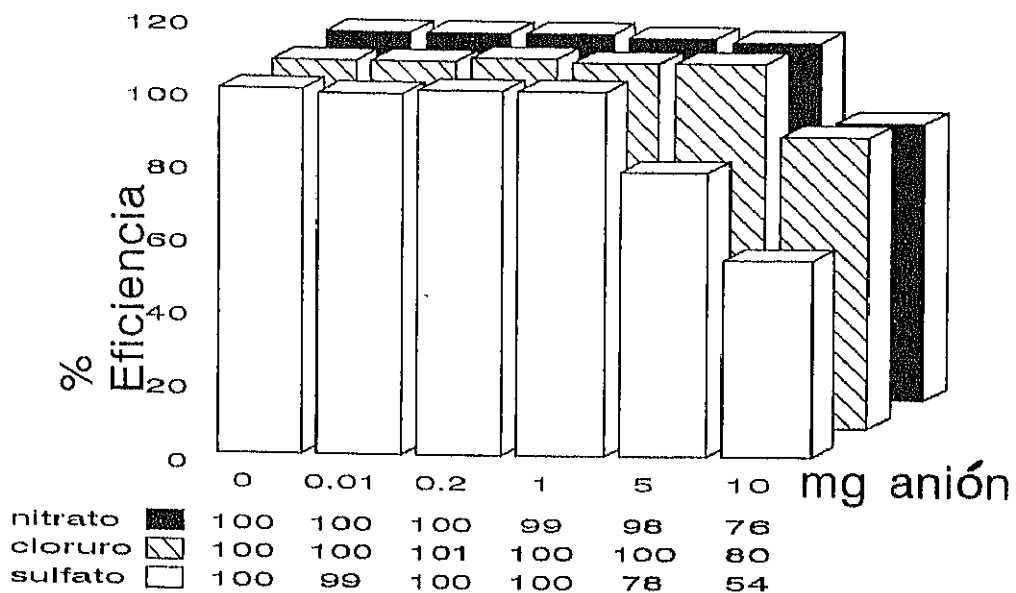
Figura 40.- Eficiencia de la preconcentración de 4 \mu\text{g L}^{-1} de As(V) en presencia de cantidades variables de Cl - , SO 4 2- y NO 3 - .
