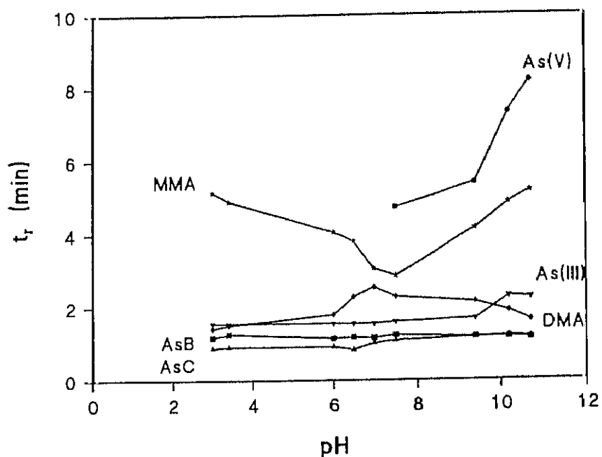
Figura 26.- Influencia del pH de la fase móvil (fosfato 1.0 \text{ mmol L}^{-1} ) en cromatografía líquida de cambio aniónico (columna IC-PAK A)-MO-HG-AAS, para la separación de seis especies de arsénico ( 200 \mu\text{g L}^{-1} de As en cada especie). Caudal: 1.0 \text{ mL min}^{-1}
