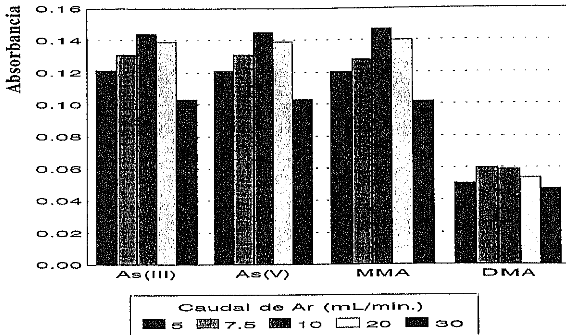
Figura 6.- Influencia del caudal de argón sobre la señal analítica de los hidruros de arsénico formados a partir de As(III), As(V), MMA y DMA. Concentración de arsénico: 200 \mu\text{g L}^{-1} .
