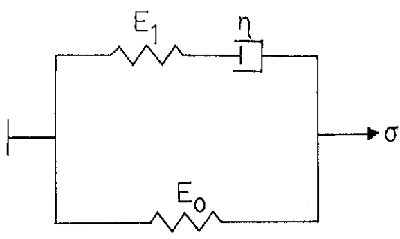
Figura 1.7.4.: Modelo o cuerpo de Maxwell Está formado por un elemento de Hooke alineado en serie con un elemento de Newton.
