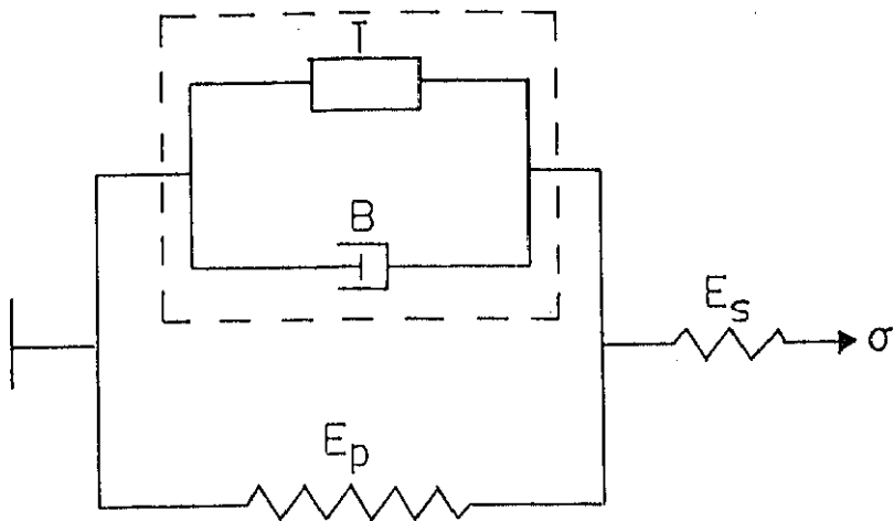
Figura 5.8.2.: Modelo de Hill del elemento contráctil El elemento contráctil (dentro del recuadro punteado), es un elemento compuesto. Esta formado por un generador de fuerza (T), alineado en paralelo con un elemento viscoso (B).
